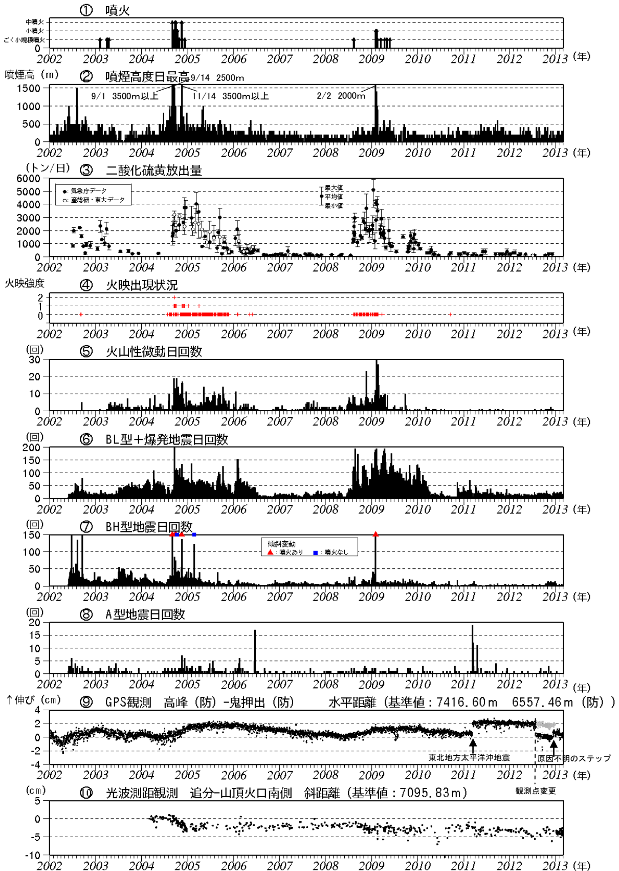
図3※ 浅間山 最近の火山活動経過図 (2002年1月1日~2013年2月28日)
