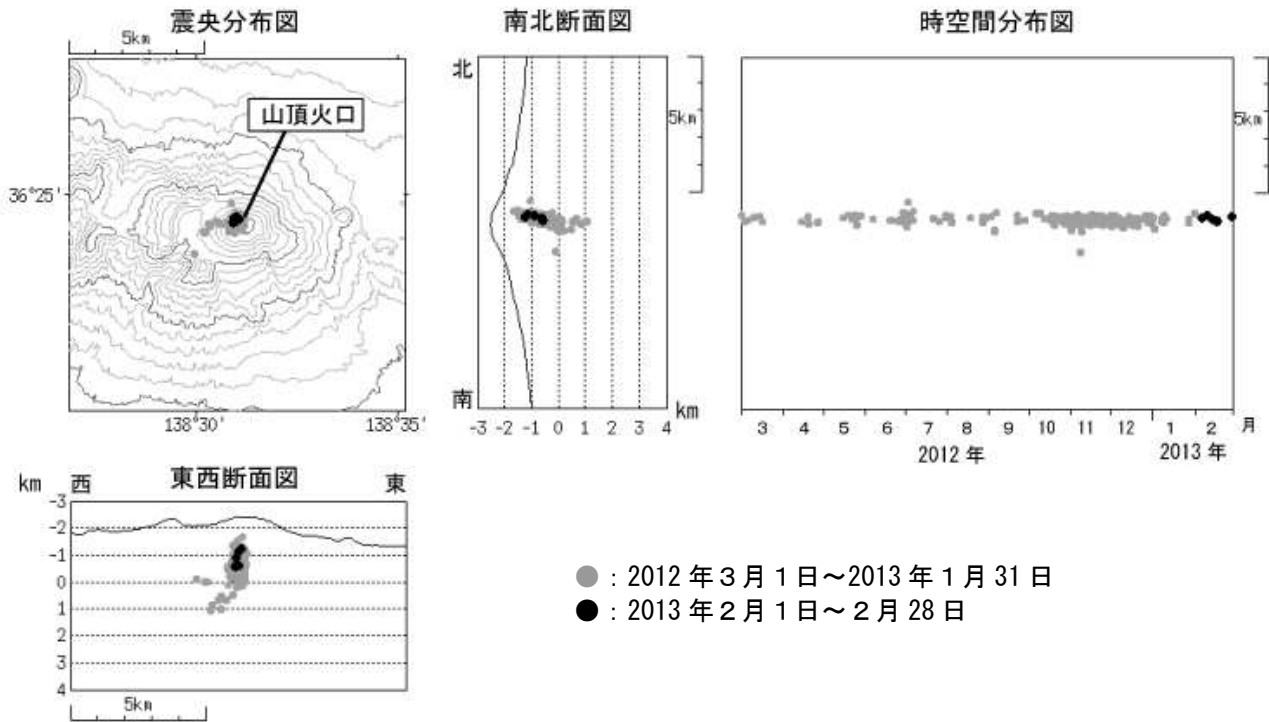
図 4※ 浅間山 震源分布図（2012 年 3 月 1 日～2013 年 2 月 28 日）
