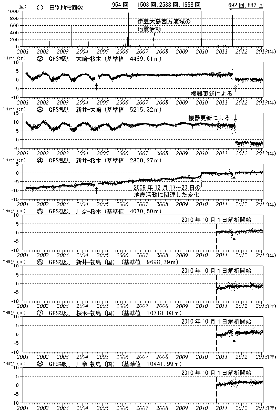
図3※ 伊豆東部火山群 最近の火山活動経過図（2001年1月～2013年1月）
