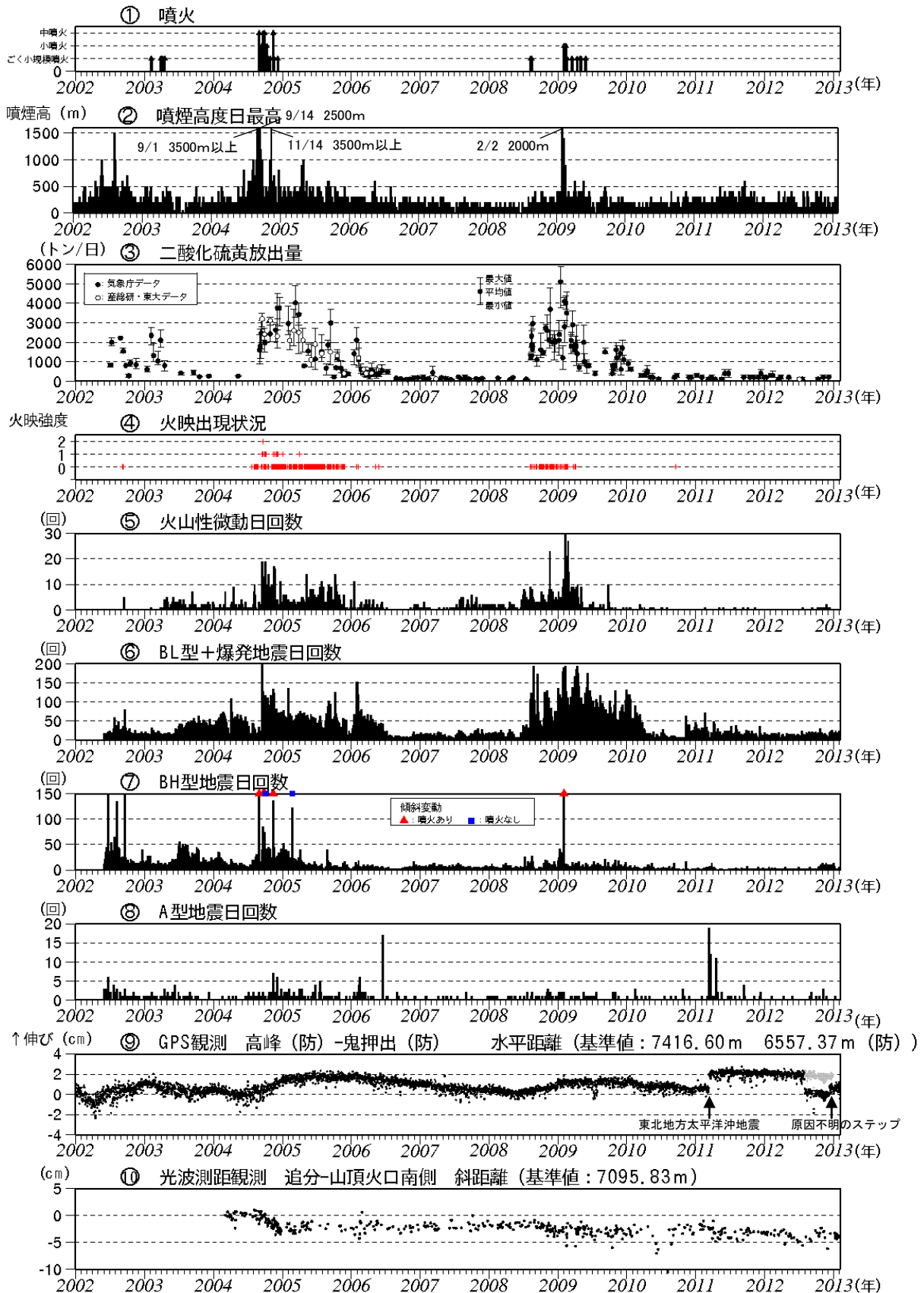
図3※ 浅間山 最近の火山活動経過図 (2002年1月1日~2013年1月31日)
