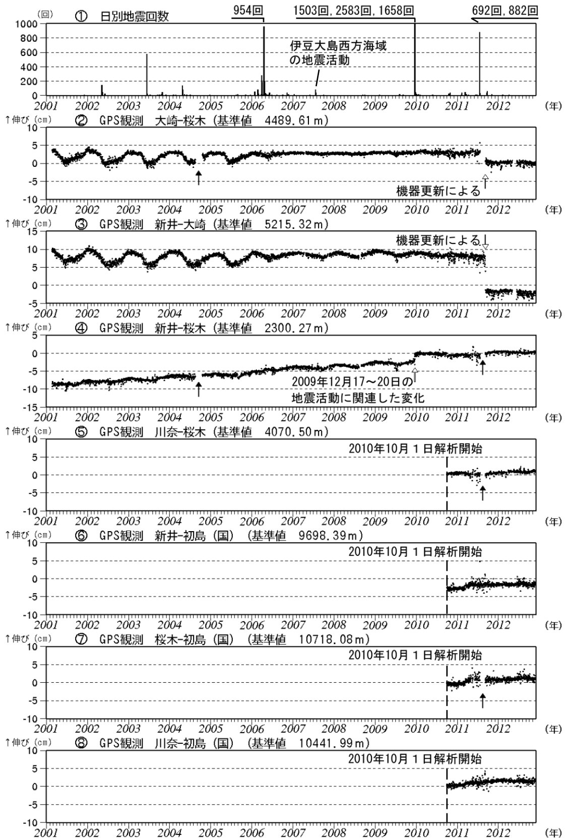
図3 伊豆東部火山群 最近の火山活動経過図（2001年1月～2012年11月）
