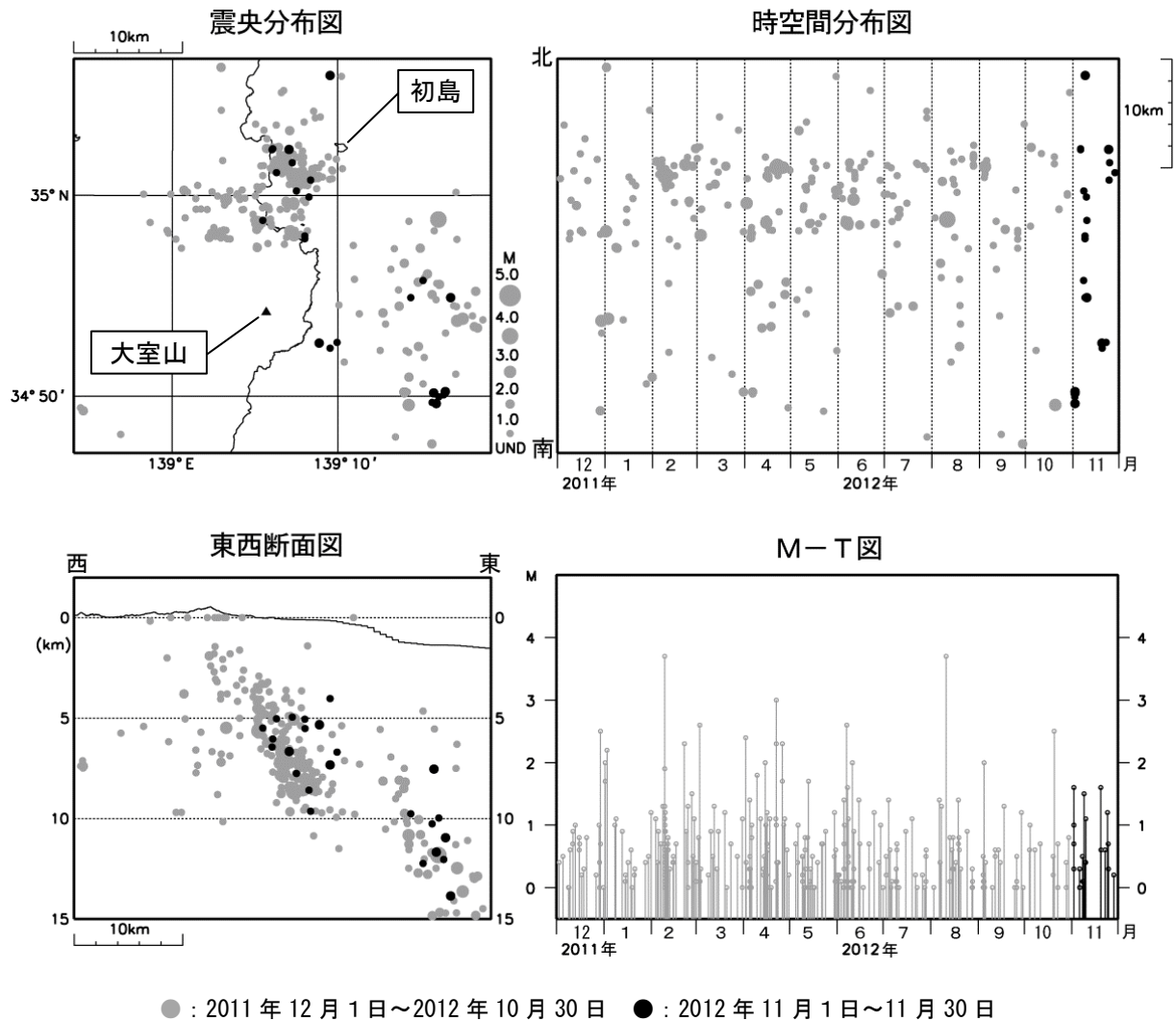
図 2※ 伊豆東部火山群 広域地震観測網による震源分布図（2011年12月1日～2012年11月30日） M（マグニチュード）は地震の規模を表します。 図中の震源要素は一部暫定値が含まれており、後日変更することがあります。
