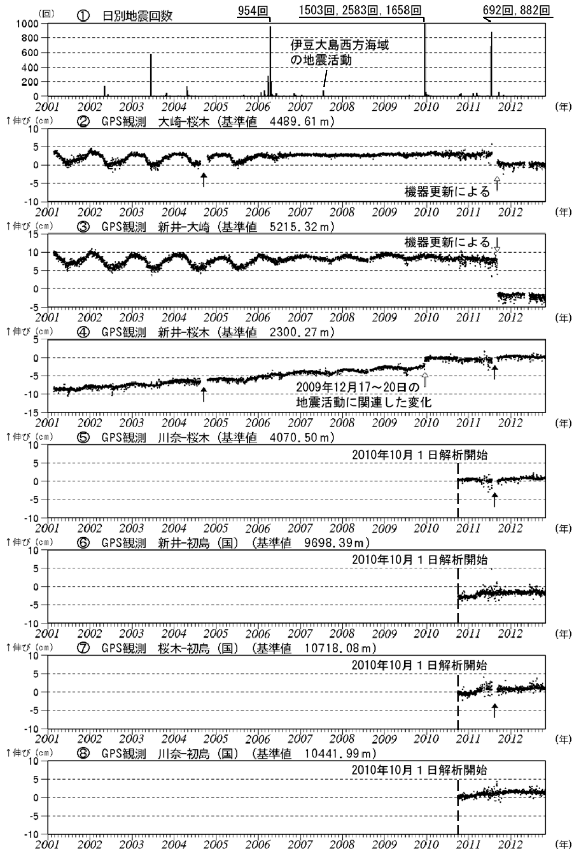
図3 伊豆東部火山群 最近の火山活動経過図（2001年1月～2012年10月）
