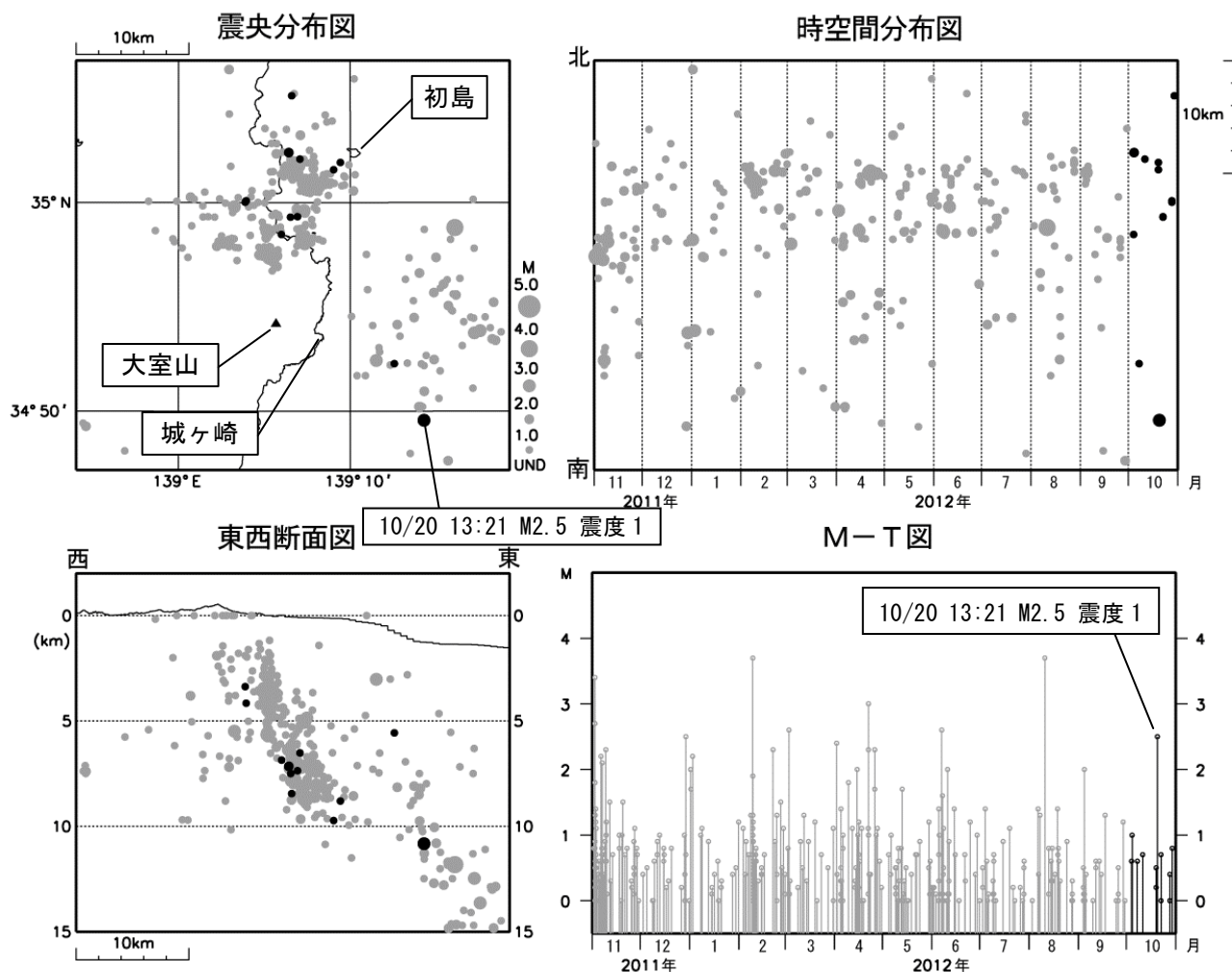
図 2※ 伊豆東部火山群 広域地震観測網による震源分布図（2011 年 11 月 1 日～2012 年 10 月 31 日）
