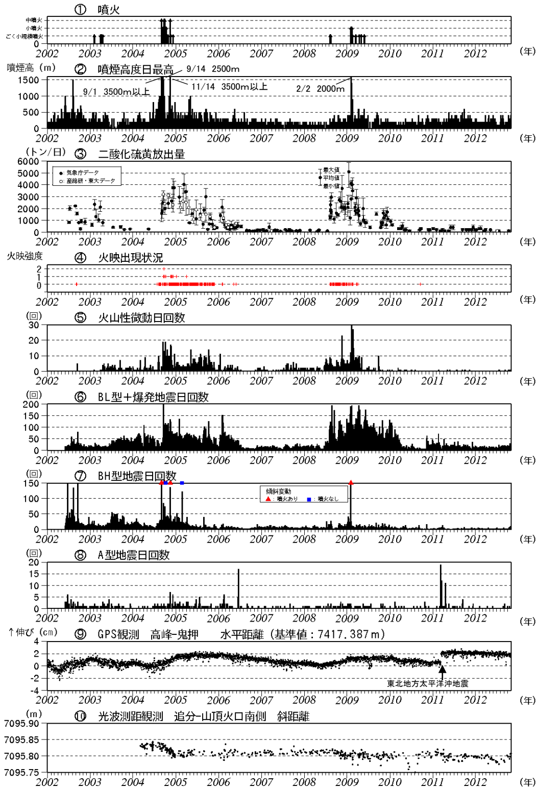
図 3※ 浅間山 最近の火山活動経過図（2002 年 1 月 1 日～2012 年 10 月 31 日）
