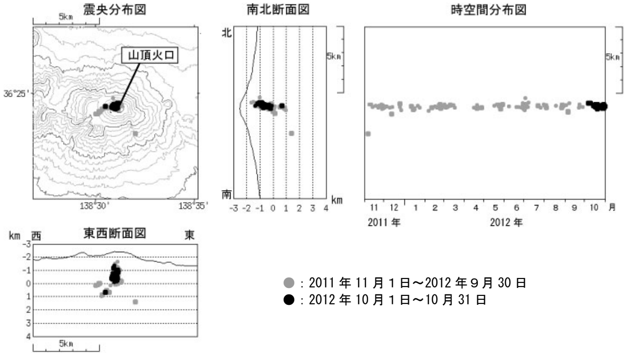
図4※ 浅間山 震源分布図（2011年11月1日～2012年10月31日）
