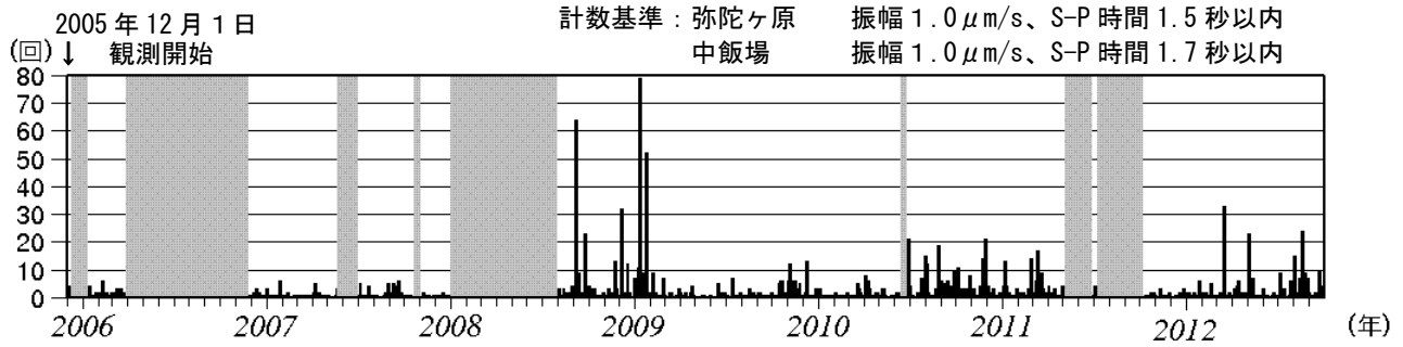
図 3 白山 日別地震回数（2005 年 12 月～2012 年 9 月）
