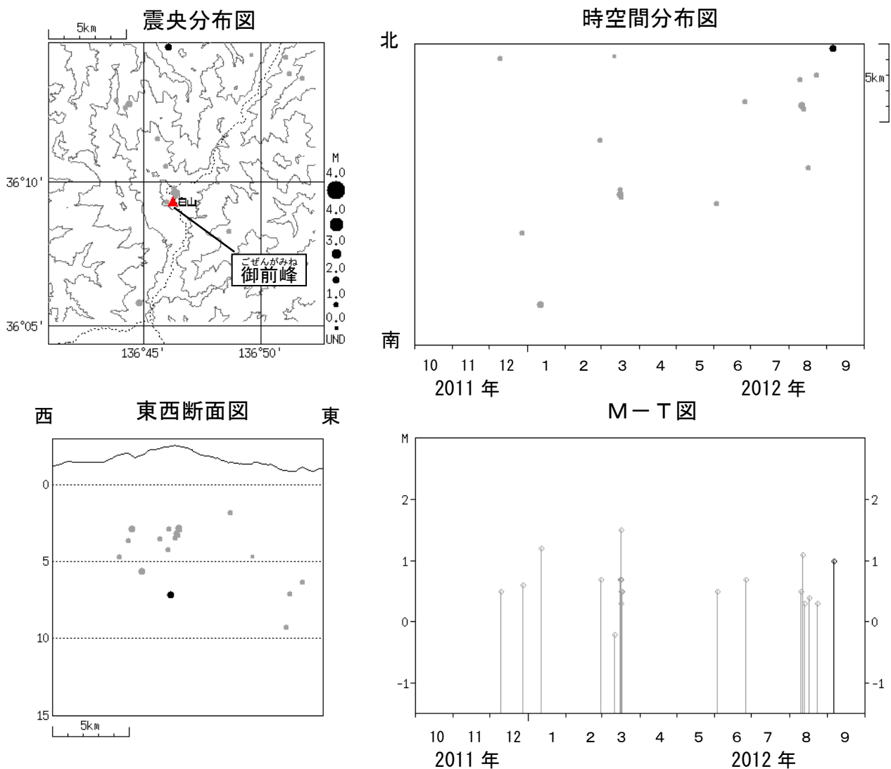
図 4 ※白山 広域地震観測網による山体・周辺の地震活動（2011 年 10 月～2012 年 9 月）
