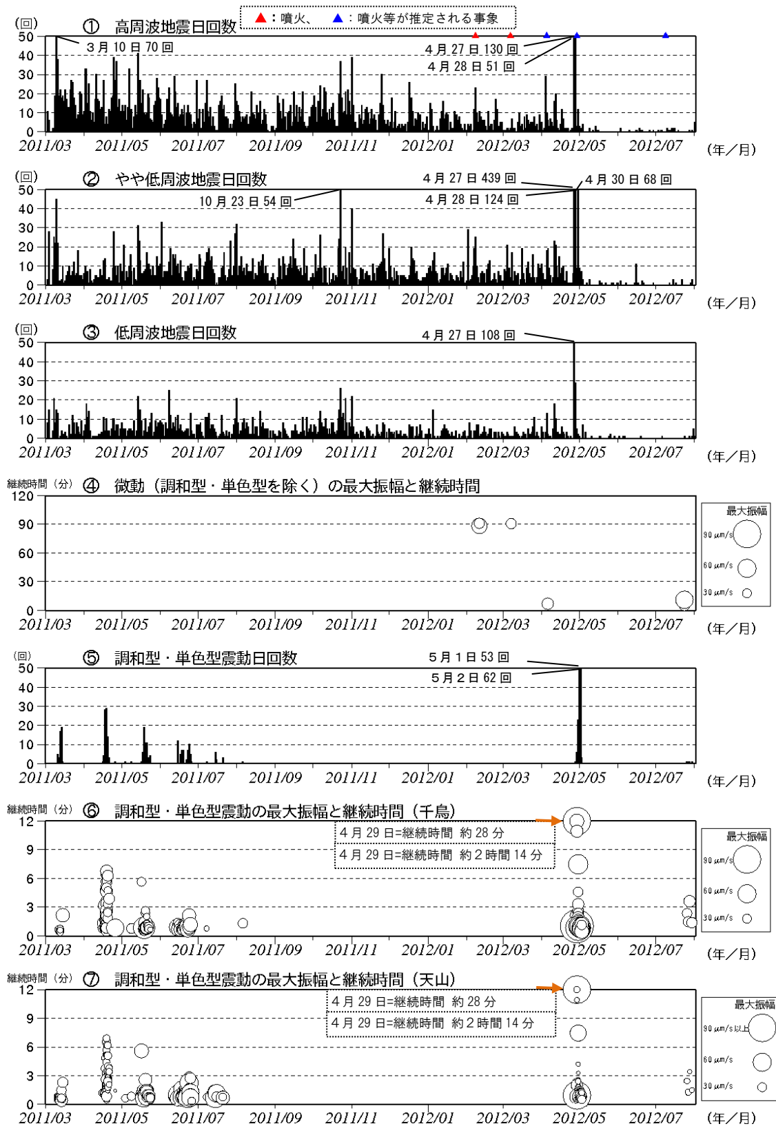
図 4※ 硫黄島 火山活動経過図（2011 年 3 月 8 日～2012 年 7 月 31 日）
