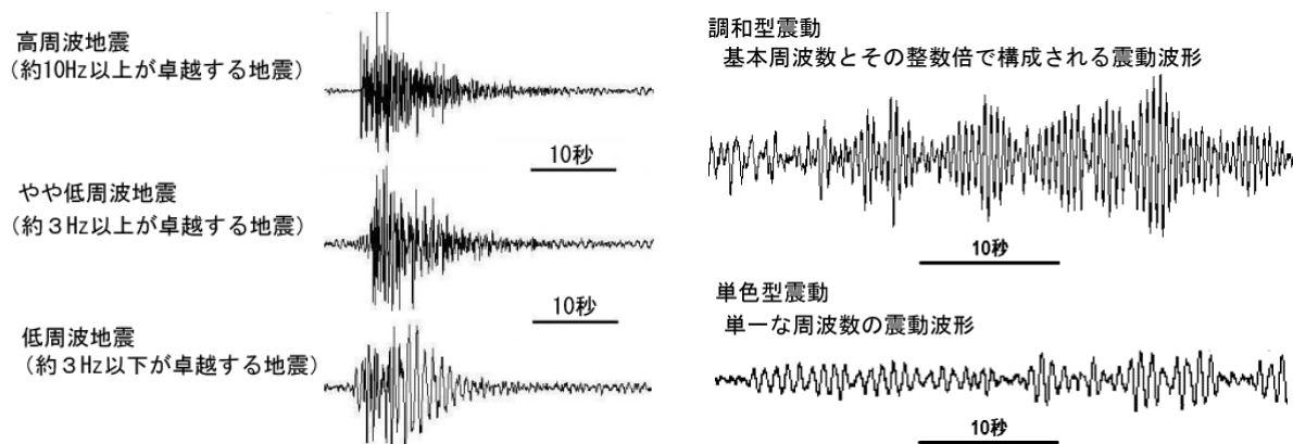
図 3 硫黄島でみられる主な火山性地震・微動（調和型震動、単色型震動）の特徴と波形例
