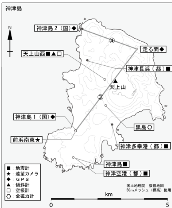
図 1 神津島 観測点配置図 GPS 基線③④は図 3 の③※④※に対応しています。
