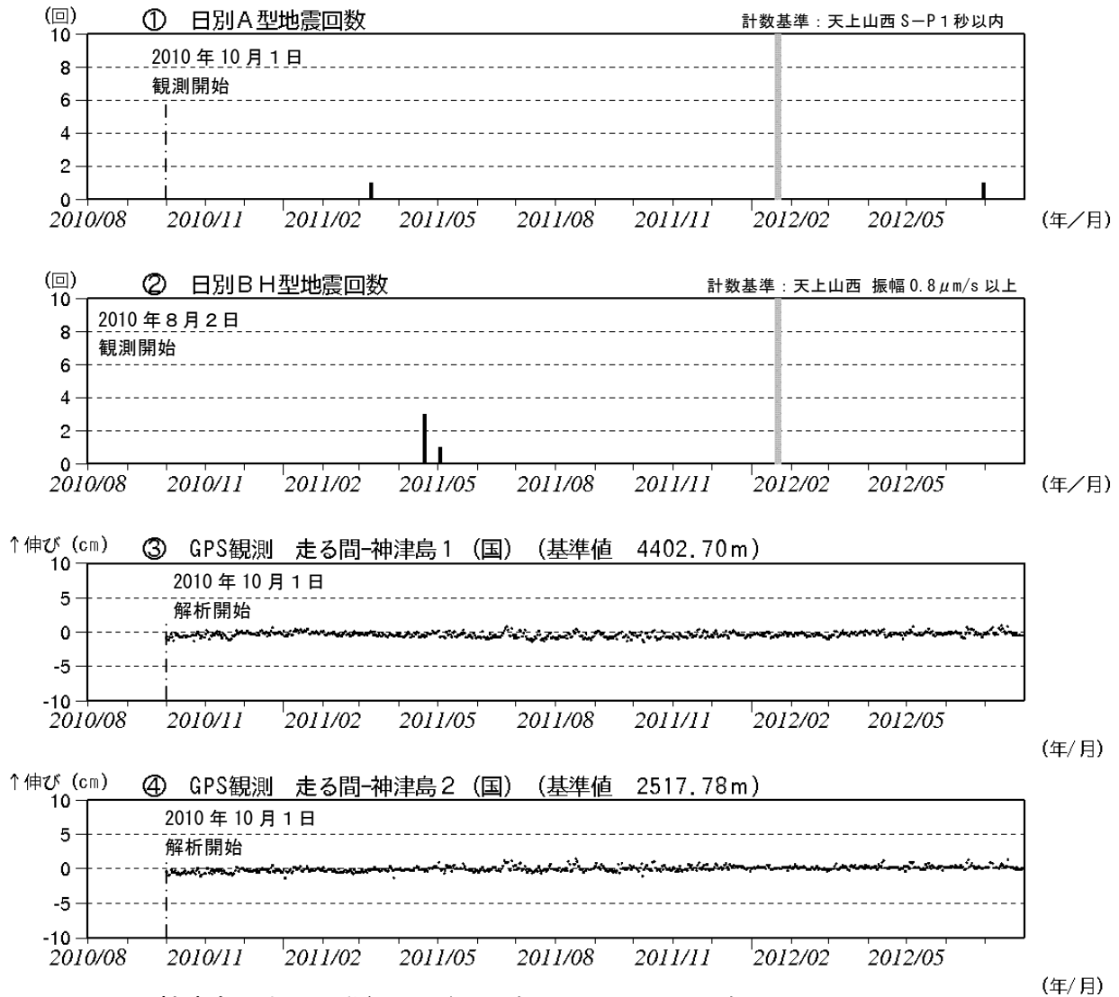
図 3 神津島 火山活動経過図(2010 年 8 月 2 日~2012 年 7 月 31 日)
