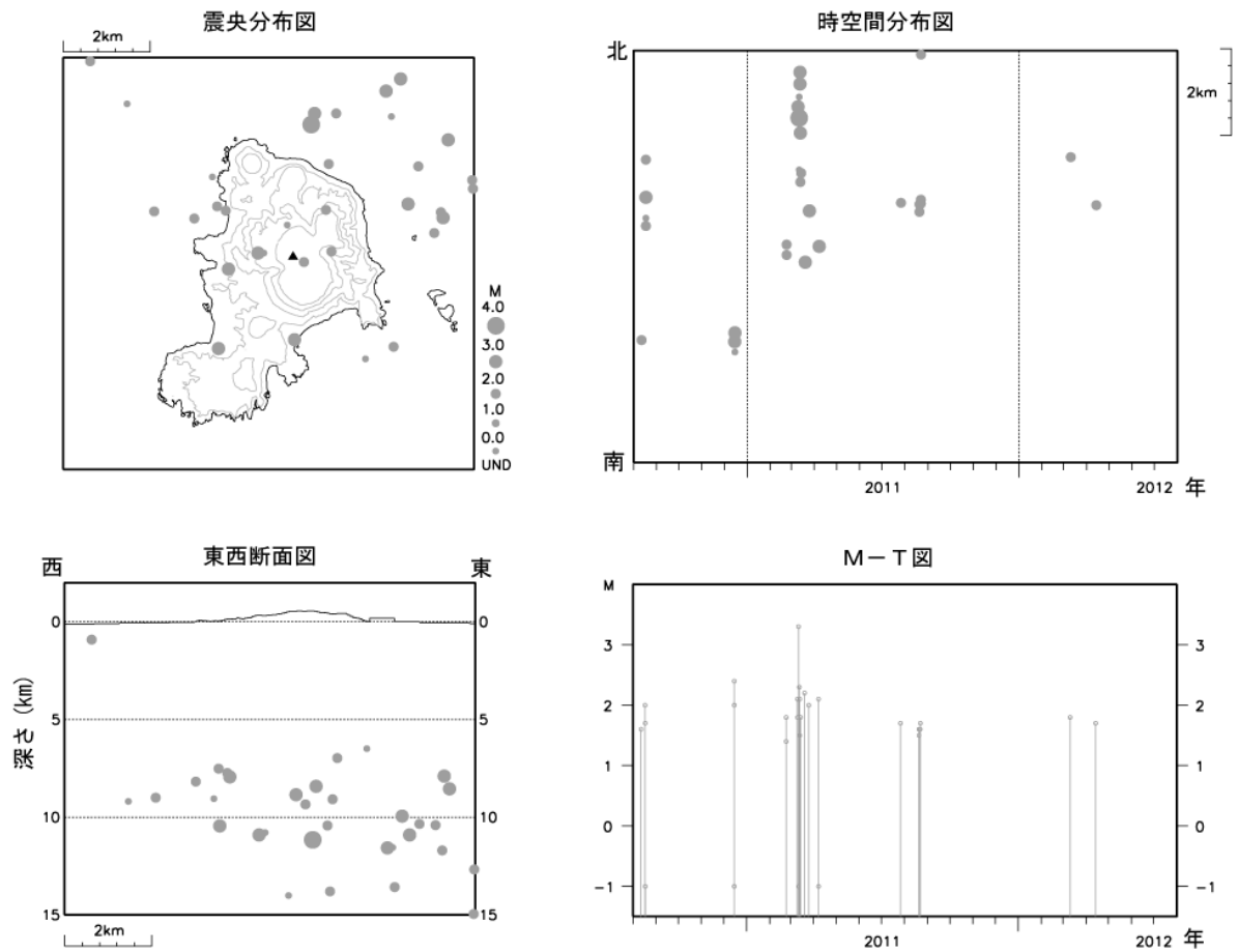
図 4 ※ 神津島 広域地震観測網による山体・周辺の地震活動（2010 年 8 月 1 日～2012 年 7 月 31 日）
