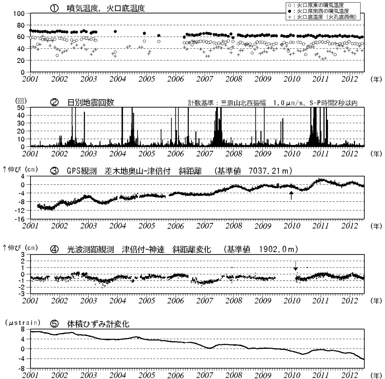
図2 伊豆大島 最近の火山活動経過図（2001年1月～2012年6月）
