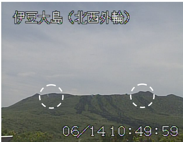
山頂部（6月14日、北西外輪遠望カメラによる） 剣ガ峰付近（6月26日、撮影方向は図6参照） 図4 伊豆大島 三原山山頂火口内及び山頂部の状況 点円内：ごく弱い噴気
