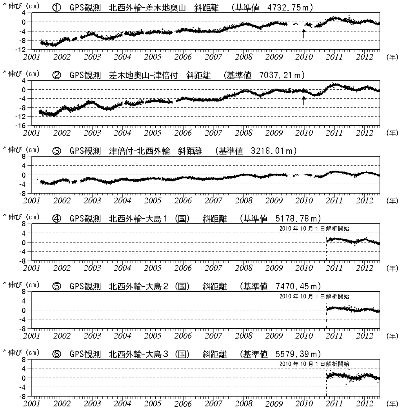
図3※ 伊豆大島 GPS 連続観測による基線長変化 (2001 年 1 月～2012 年 6 月) (国) : 国土地理院 2010 年 10 月以降のデータについては、電離層の影響を補正する等、解析方法を改良しています。 ①～③、及び④*～⑥*は図8のGPS基線①～⑥に対応しています。 グラフの空白部分は欠測。①②の矢印は差木地奥山支柱工事による変動。
