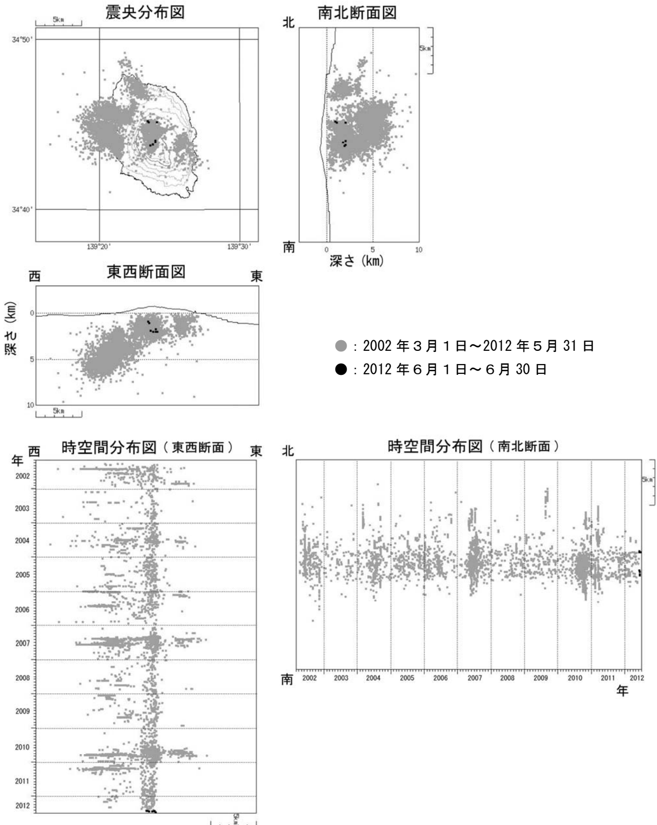
図 7※ 伊豆大島 震源分布図 (2002 年 3 月 1 日 ~ 2012 年 6 月 30 日)
