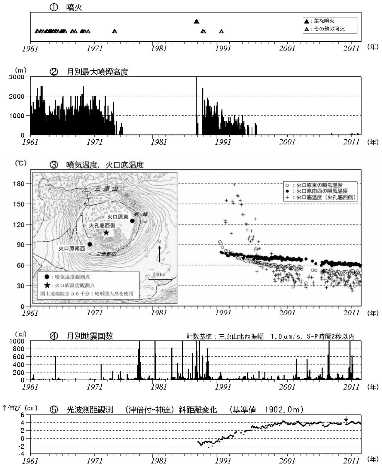
図 1 伊豆大島 長期間の火山活動経過図 (1961 年 1 月～2012 年 6 月)
