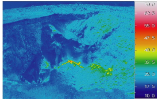
2012年6月26日14時30分撮影
