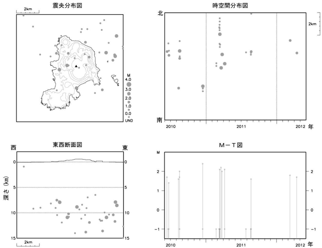
図 4※ 神津島 広域地震観測網による山体・周辺の地震活動（2010 年 6 月 1 日～2012 年 5 月 31 日）
