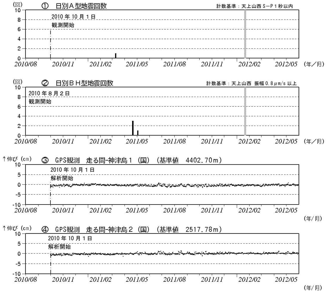
図 3 神津島 火山活動経過図(2010 年 8 月～2012 年 5 月)
