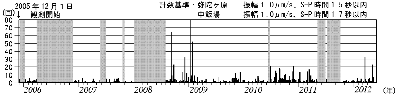
図3 白山 日別地震回数 (2005年12月~2012年5月)
