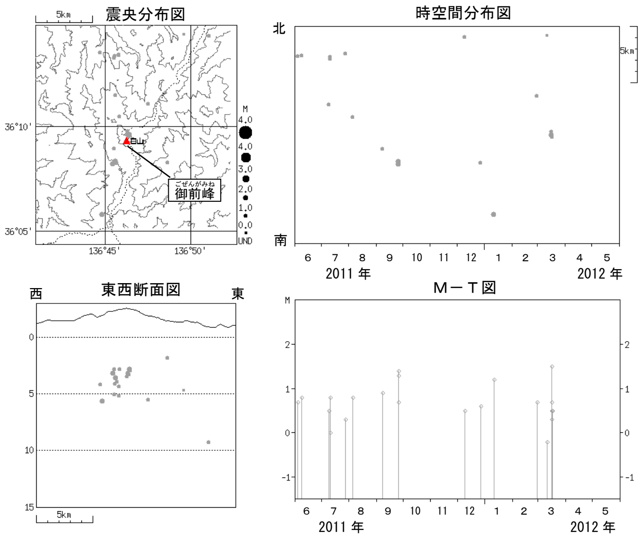
図4※白山 広域地震観測網による山体・周辺の地震活動 (2011年6月~2012年5月)
