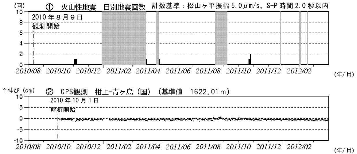
図 2 青ヶ島 火山活動の推移（2010 年 8 月 9 日～2012 年 4 月 30 日）
