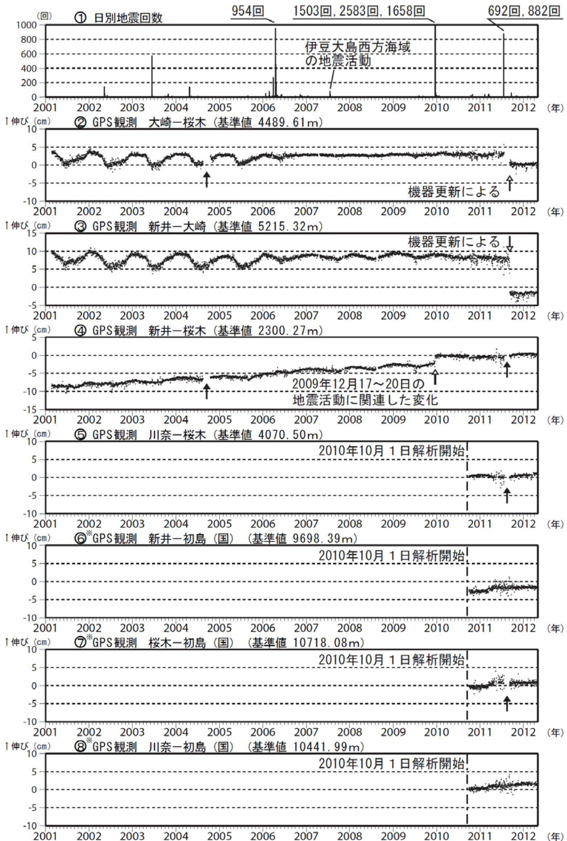
図3 伊豆東部火山群 最近の火山活動経過図（2001年1月～2012年4月）
