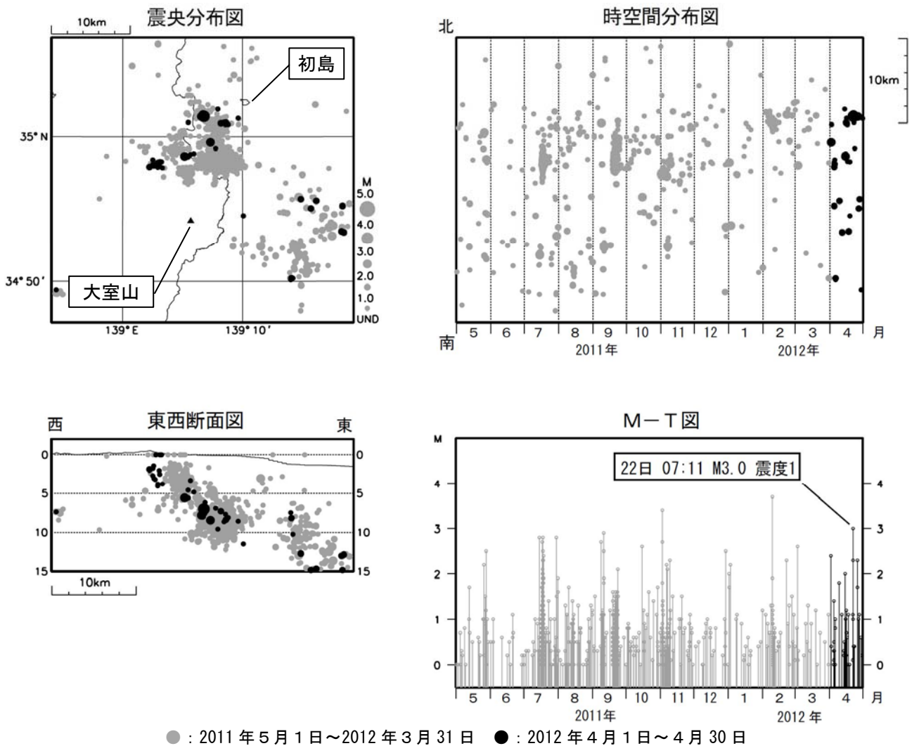
図2※ 伊豆東部火山群 広域地震観測網による震源分布図（2011年5月1日～2012年4月30日） M（マグニチュード）は地震の規模を表します。 図中の震源要素は一部暫定値が含まれており、後日変更することがあります。
