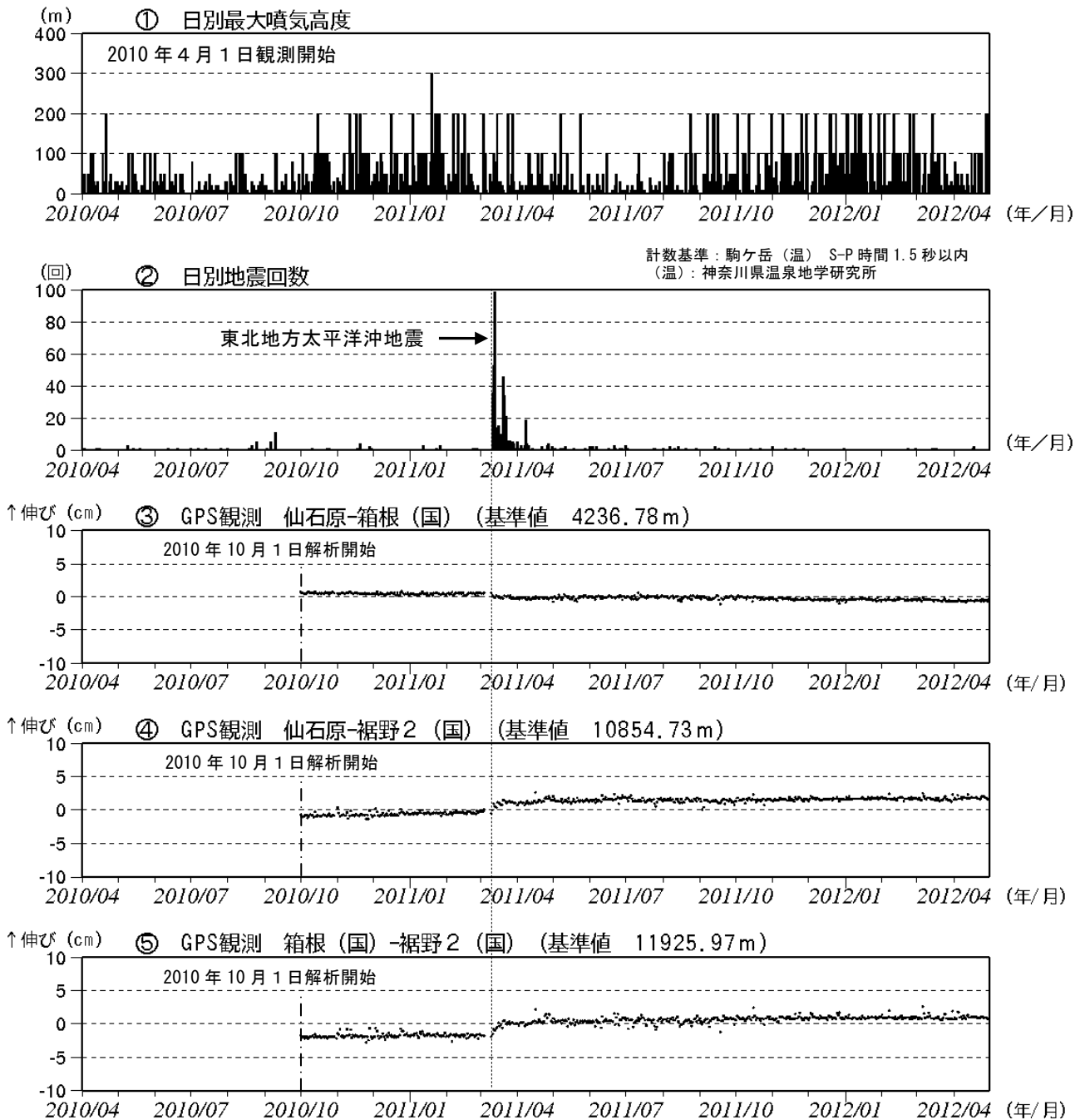
図3 箱根山 火山活動経過図（2010年4月1日～2012年4月30日）
