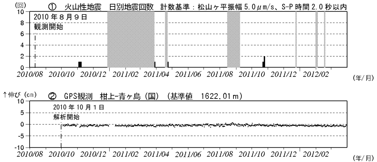
図 2 青ヶ島 火山活動の推移（2010 年 8 月 9 日～2012 年 3 月 31 日）
