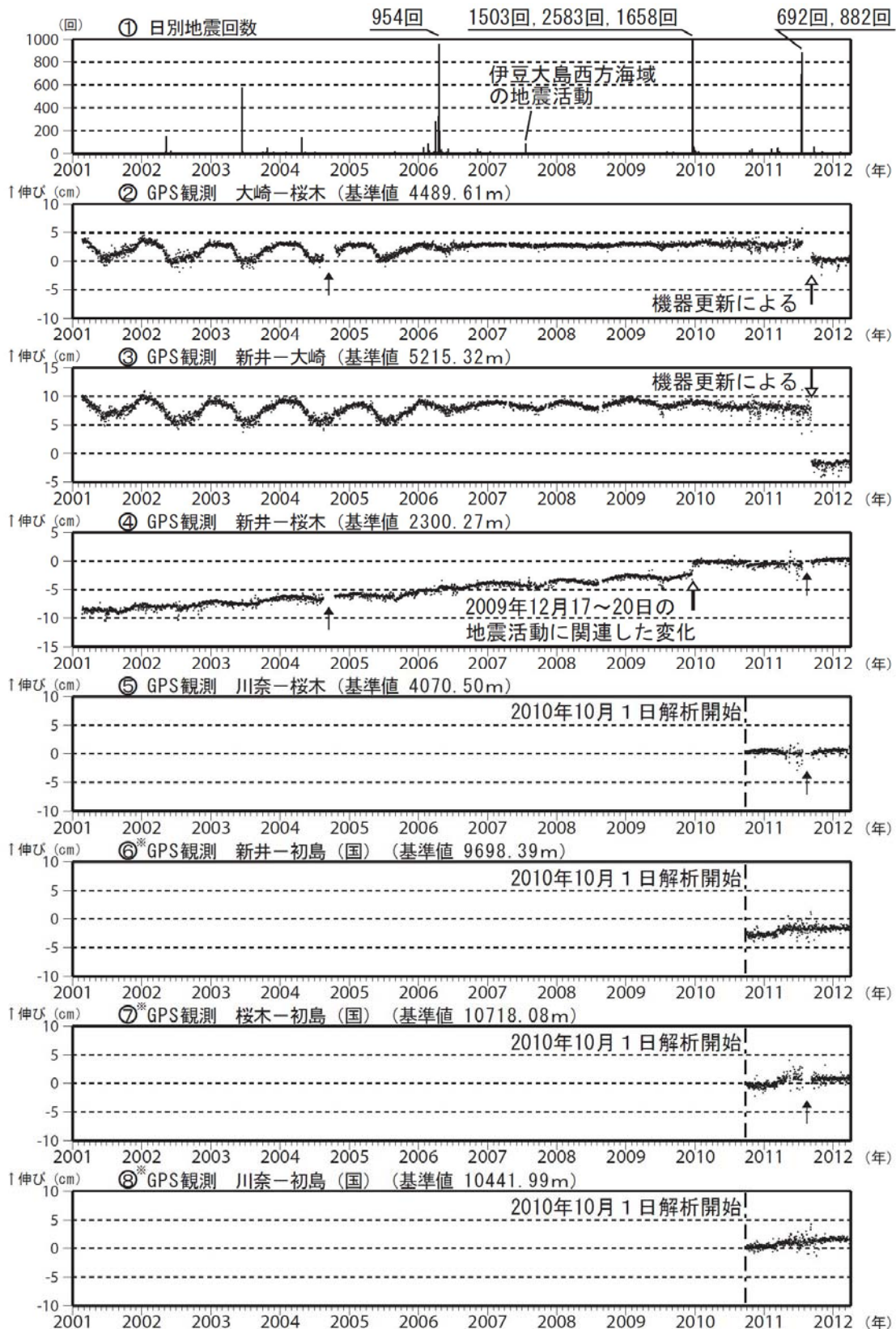
図3 伊豆東部火山群 最近の火山活動経過図（2001年1月～2012年3月）
