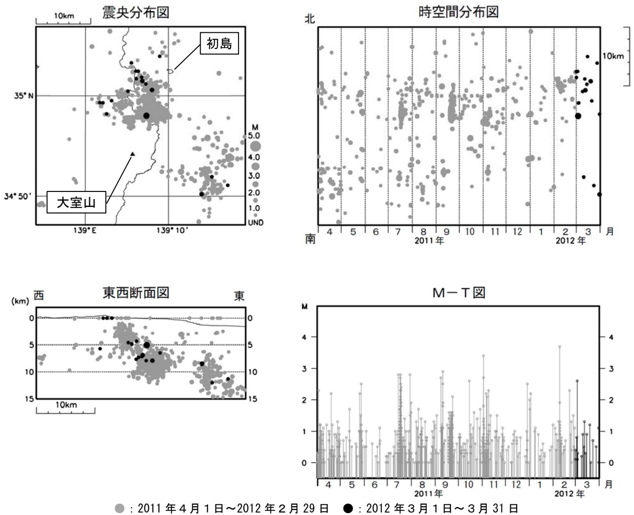
図 2※ 伊豆東部火山群 広域地震観測網による震源分布図（2011 年 4 月 1 日～2012 年 3 月 31 日） M（マグニチュード）は地震の規模を表します。 図中の震源要素は一部暫定値が含まれており、後日変更することがあります。
