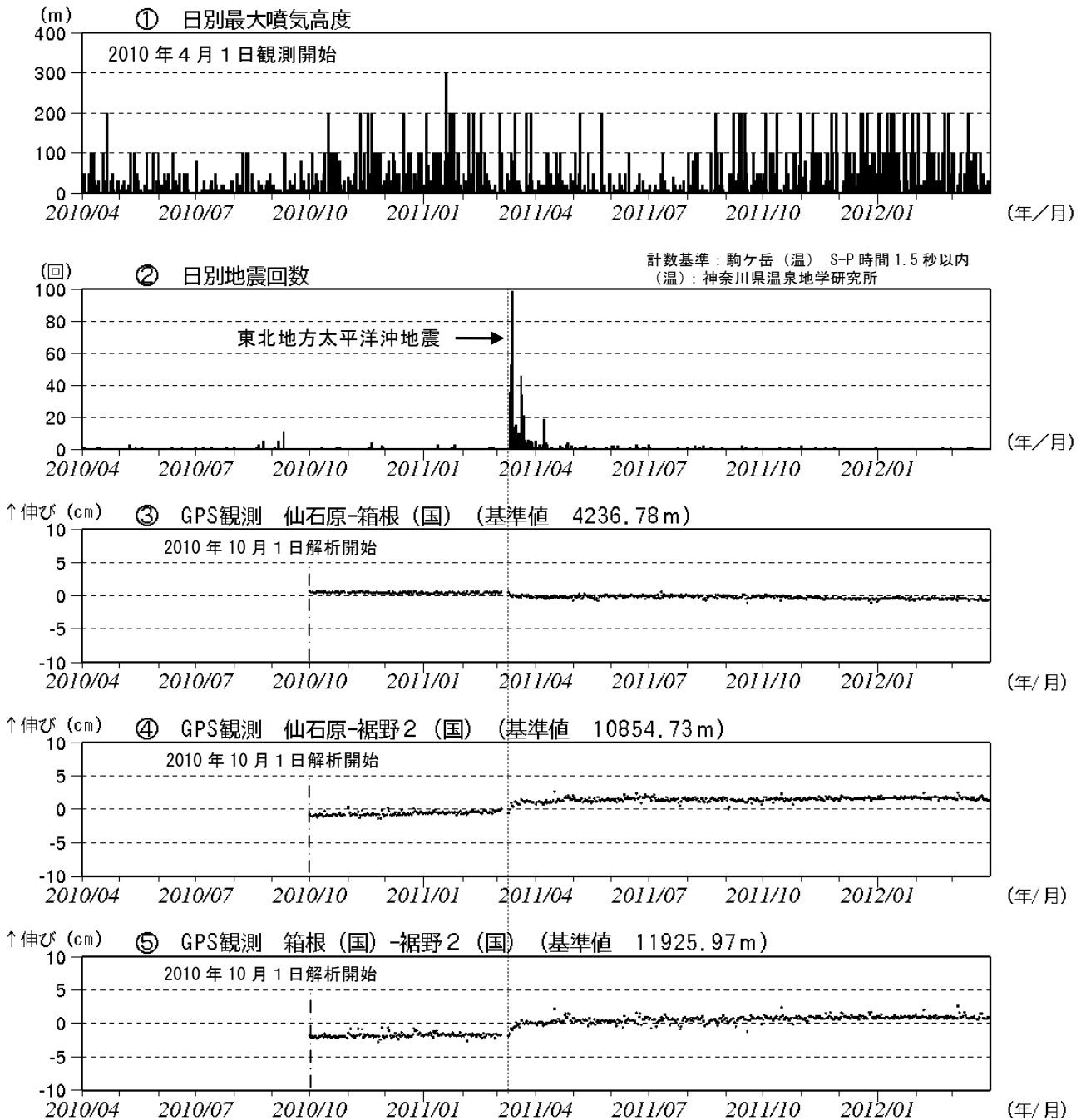
図3 箱根山 火山活動経過図（2010年4月1日～2012年3月31日）
