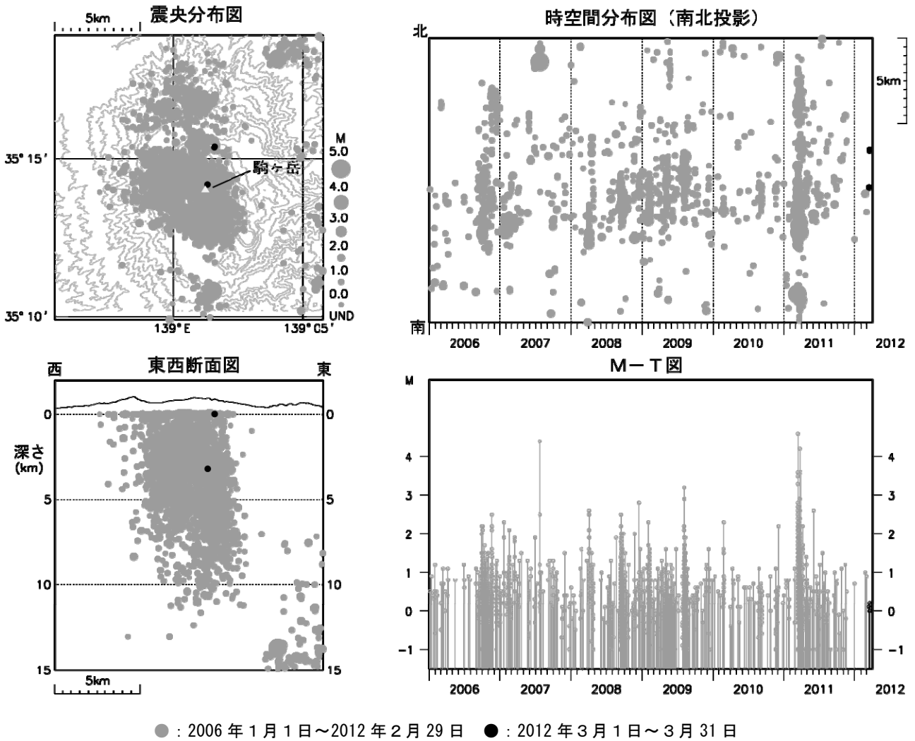
図 4※ 箱根山 広域地震観測網による山体・周辺の震源分布図（2006 年 1 月 1 日～2012 年 3 月 31 日） M（マグニチュード）は地震の規模を表します。 今期間、震源が決定された地震は少なく、地震活動は静穏に経過しました。 図中の震源要素は一部暫定値が含まれており、後日変更することがあります。
