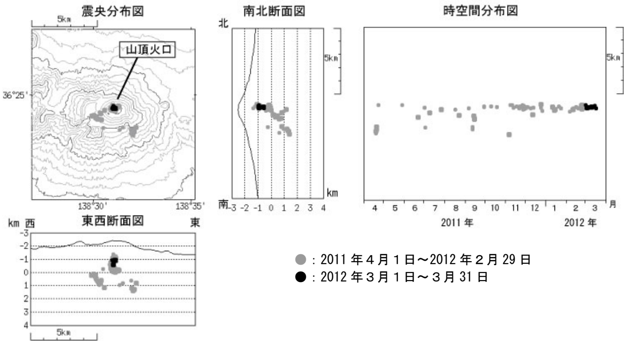
図 4 ※ 浅間山 震源分布図（2011 年 4 月 1 日～2012 年 3 月 31 日）
