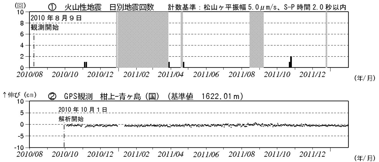
図 2 青ヶ島 火山活動の推移（2010 年 8 月 9 日～2012 年 1 月 31 日）
