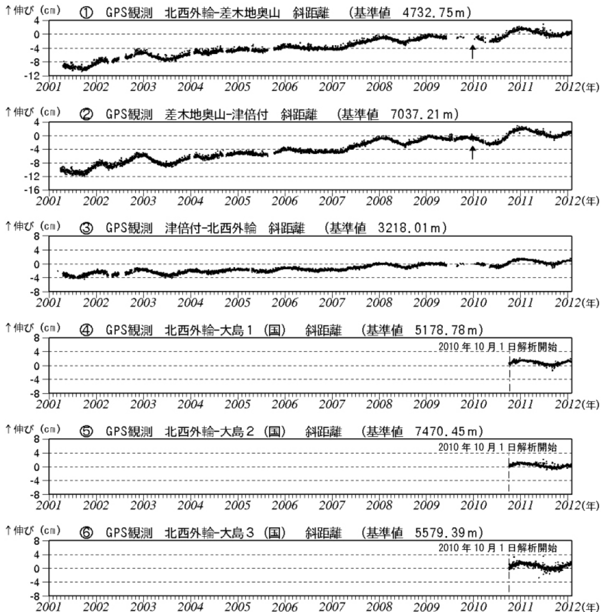
図 4 ※ 伊豆大島 GPS 連続観測による基線長変化 (2001 年 1 月～2012 年 1 月) (国): 国土地理院 2010 年 10 月以降のデータについては、電離層の影響を補正する等、解析方法を改良しています。 また、掲載する基線を一部変更しました。 ①～③、及び④※～⑥※は図 6 の GPS 基線①～⑥に対応しています。 グラフの空白部分は欠測。①②の矢印は差木地奥山支柱工事による変動。
