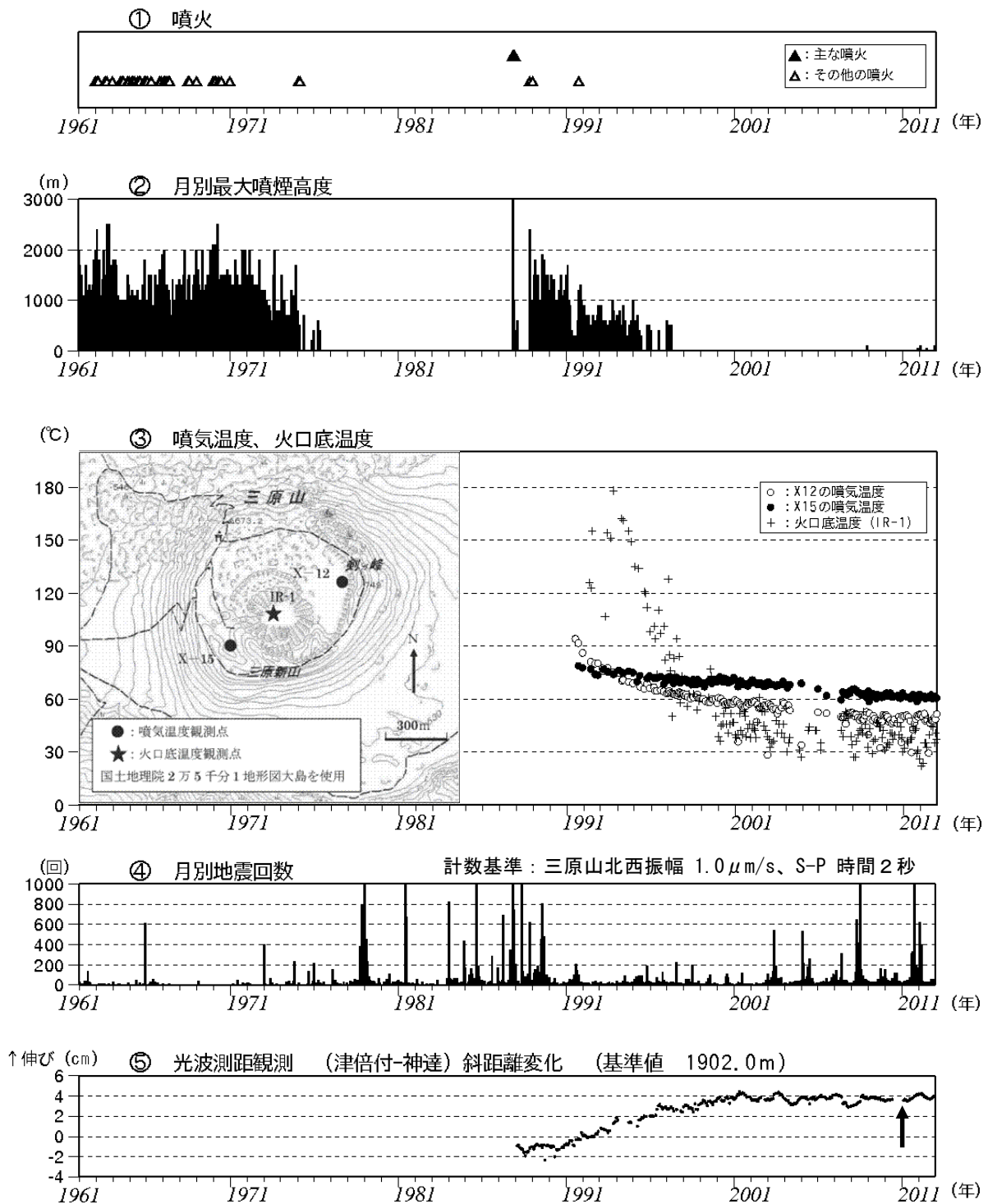
図 2 伊豆大島 長期間の火山活動経過図 (1961 年 1 月～2012 年 1 月)
