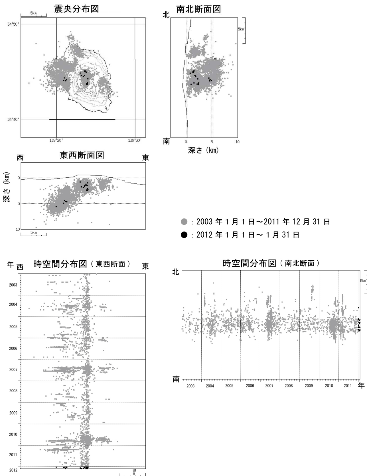
図 5※ 伊豆大島 震源分布図 (2003 年 1 月 1 日～2012 年 1 月 31 日)
