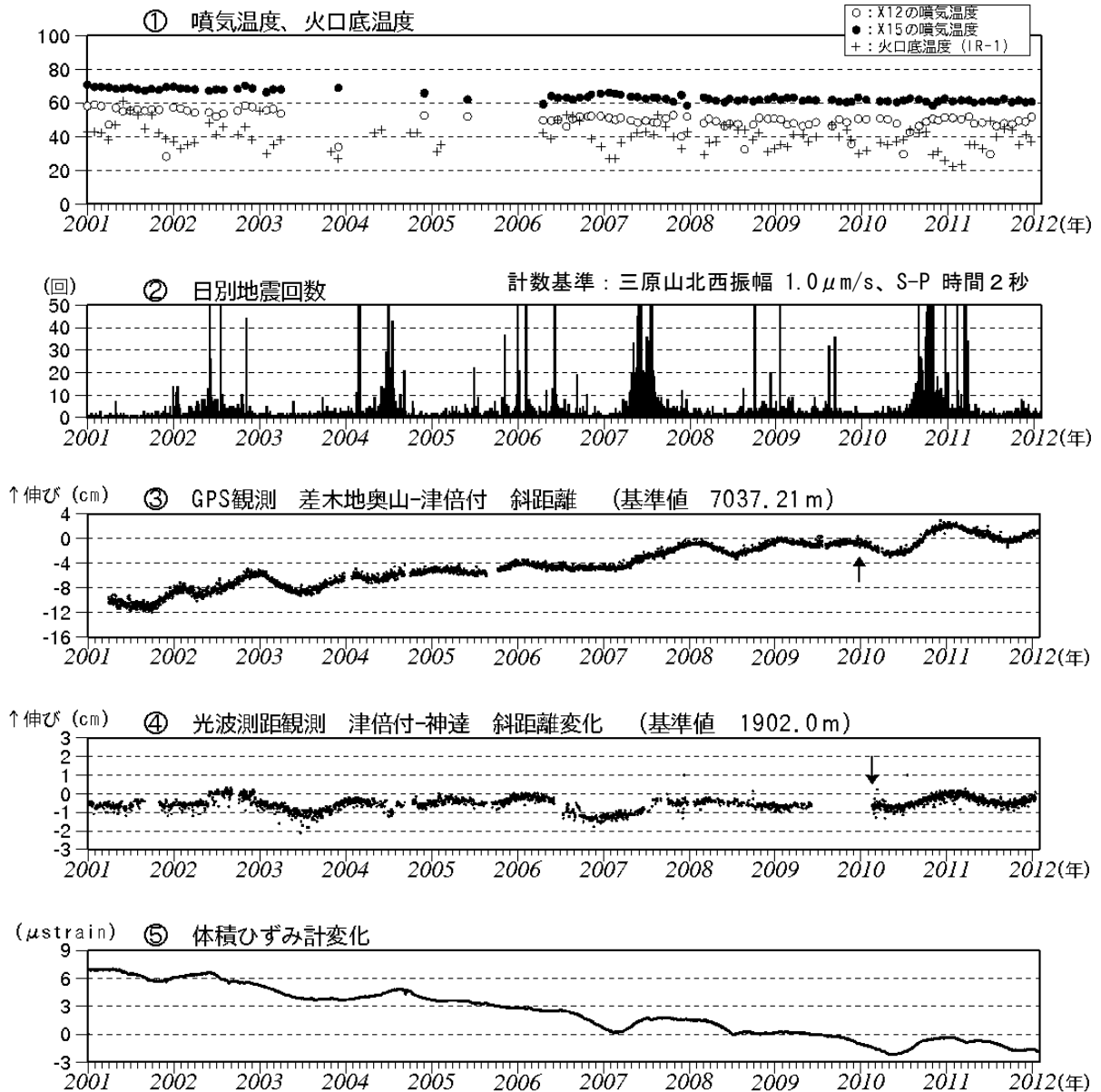
図3 伊豆大島 最近の火山活動経過図 (2001年1月～2012年1月)
