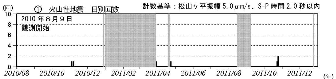
図 3 青ヶ島 火山性地震日別回数（2010 年 8 月 9 日～2011 年 12 月 31 日） 図の灰色部分は機器障害のため欠測
