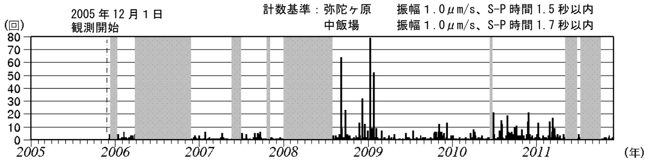
図 3 白山 日別地震回数（2005 年 12 月～2011 年 11 月）
