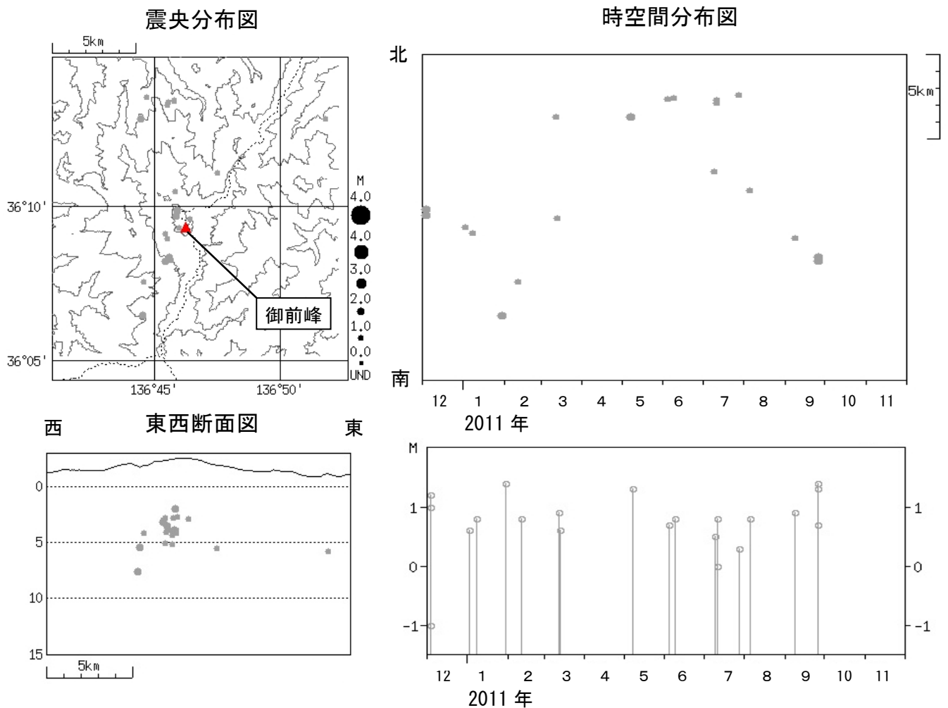
図 4 ※ 広域地震観測網による白山周辺の地震活動（2010 年 12 月～2011 年 11 月）
