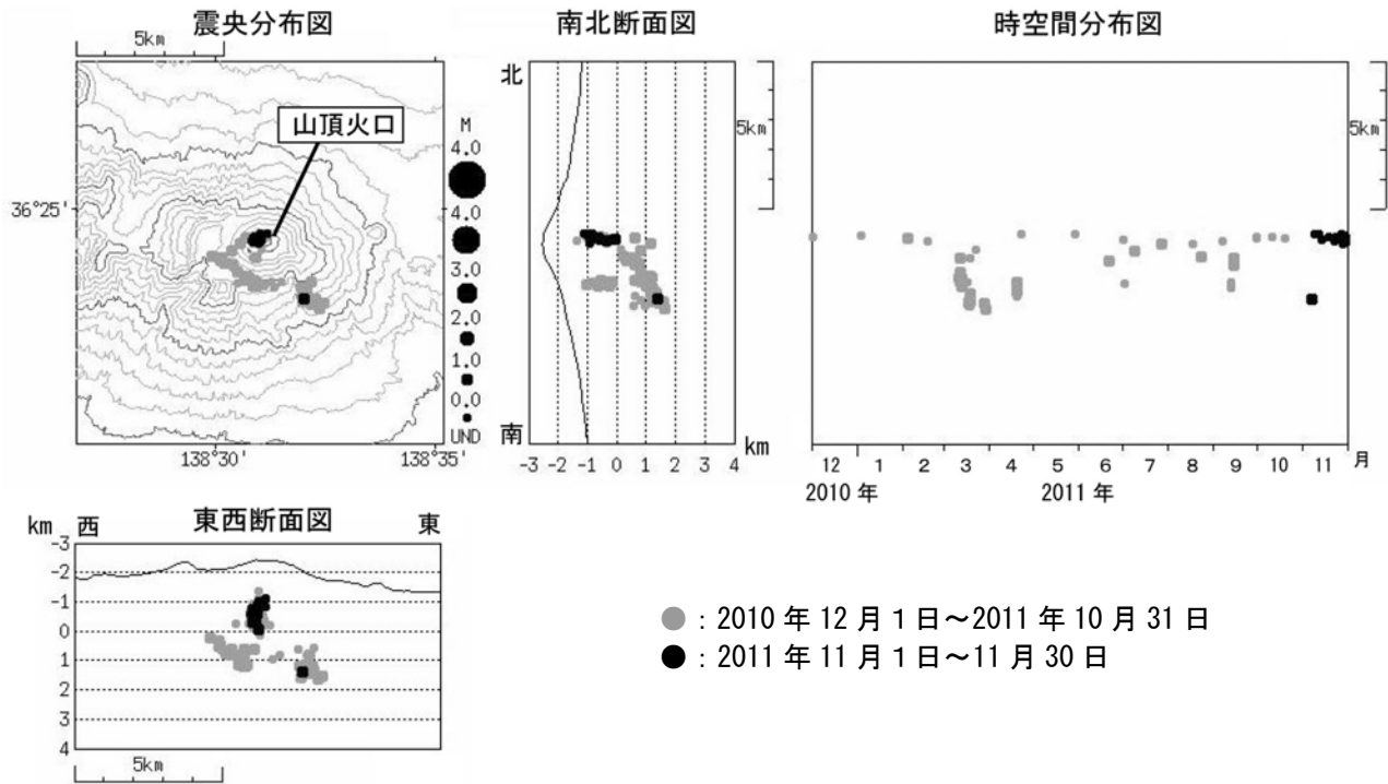
図 6※ 浅間山 震源分布図（2010 年 12 月 1 日～2011 年 11 月 30 日）
