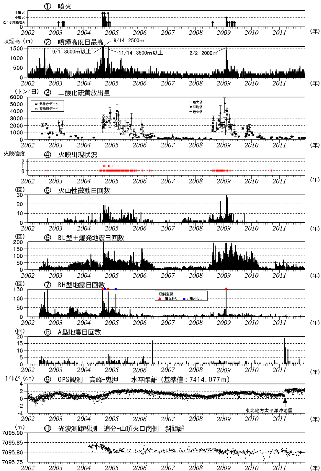
図 5 ※ 浅間山 最近の火山活動の推移 (2002 年 1 月 1 日～2011 年 11 月 30 日)
