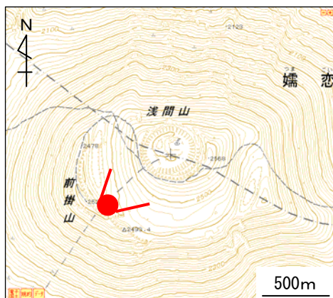
図 3 浅間山 山頂火口の状況及び赤外熱映像装置による地表面温度分布 1)
