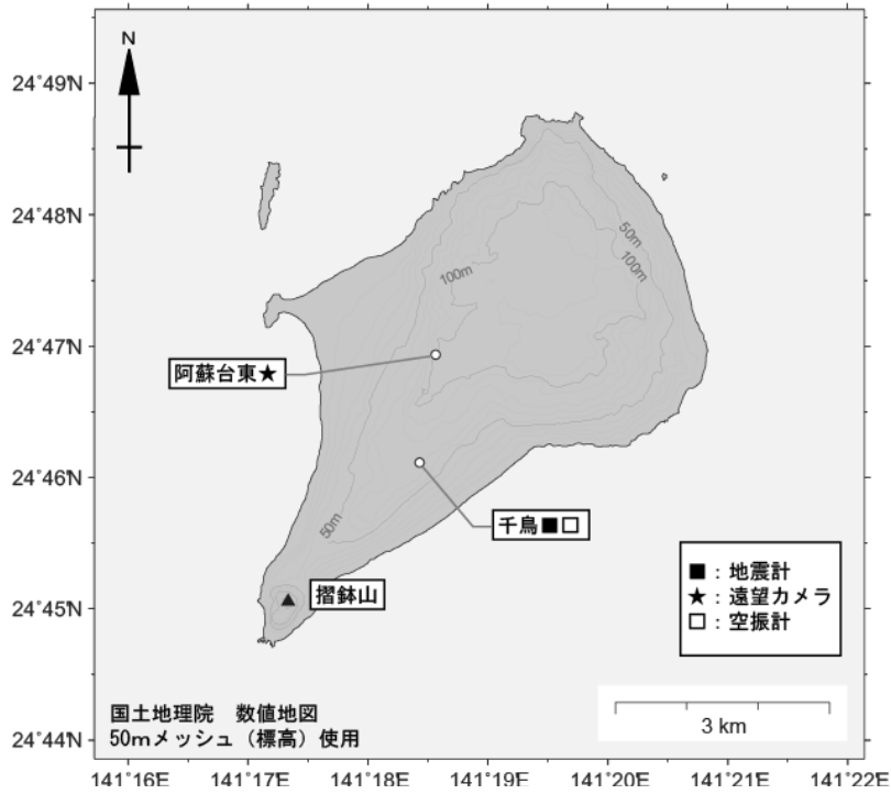
図1 硫黄島 気象庁の観測点配置図(小さな白丸は観測点位置を示しています)運用開始前の観測点も含まれます。
