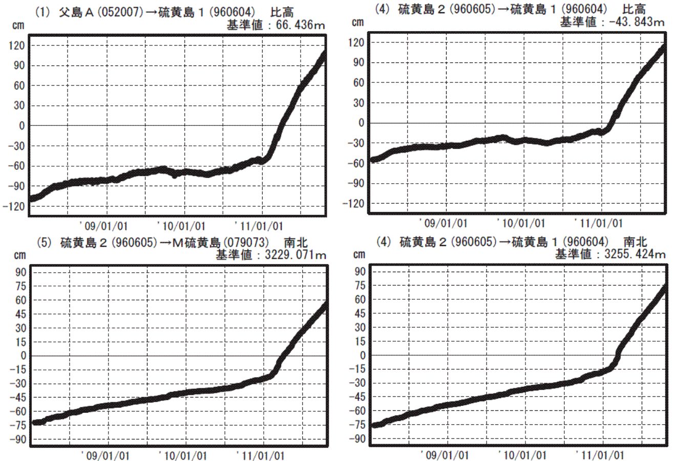
図3 硫黄島 国土地理院によるGPS観測結果 1) (2008年1月1日~2011年10月26日)
