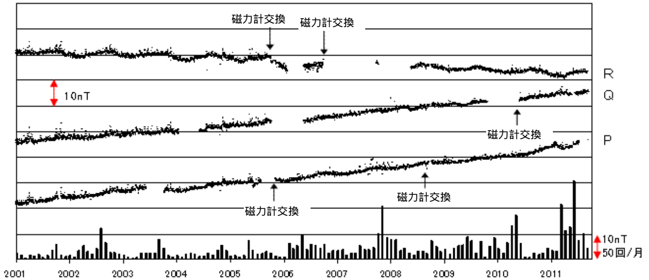
図4 草津白根山 全磁力連続観測 1) による全磁力値の変化(2001年1月~2011年9月)
