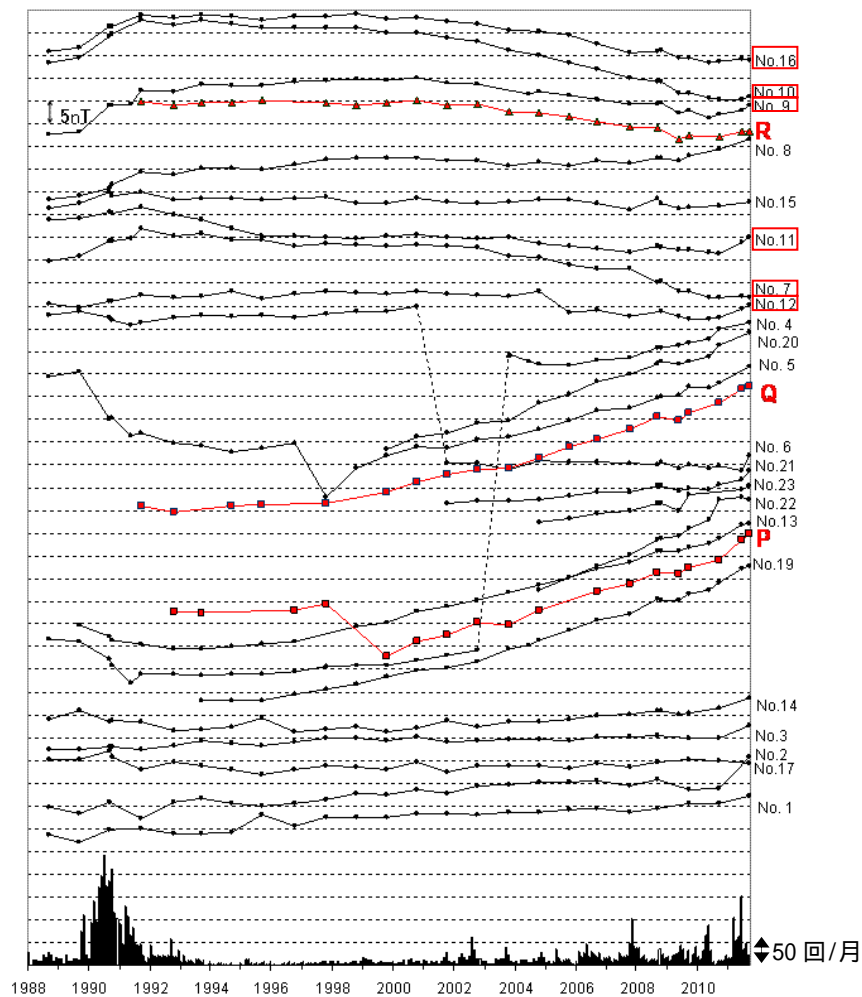
図3 草津白根山 全磁力繰り返し観測 1) による全磁力値の変化(1988年1月~2011年9月)
