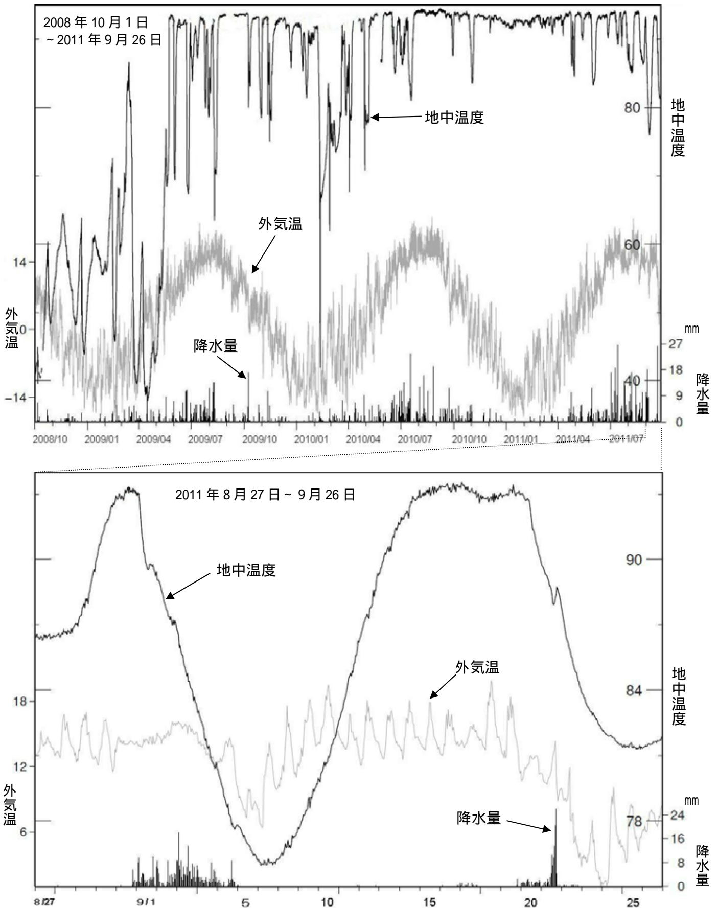
図6 草津白根山 湯釜火口内北東部の噴気地帯 地中温度、外気温と降水量(湯釜内)
