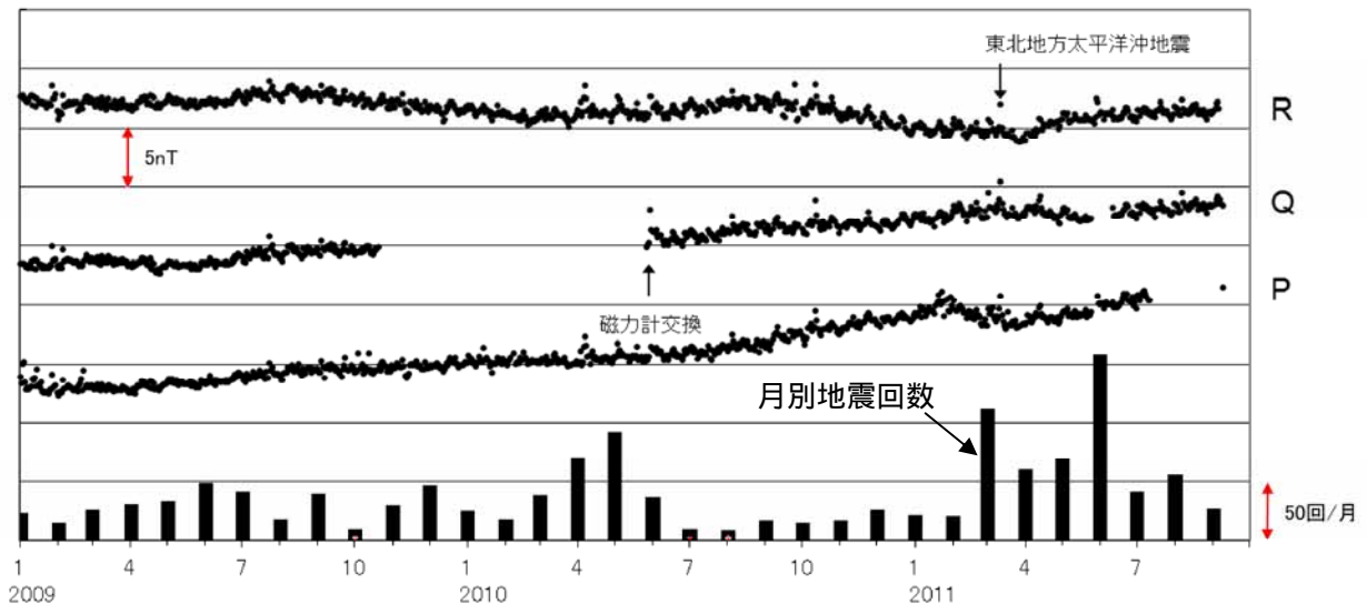
図5 草津白根山 全磁力連続観測 1) による全磁力値の変化(2009年1月~2011年9月)
