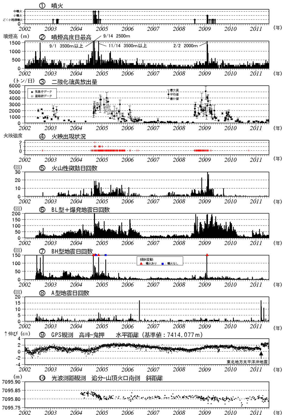
図 3※ 浅間山 最近の火山活動の推移（2002 年 1 月 1 日～2011 年 6 月 30 日）
