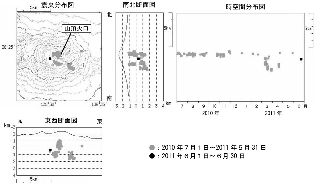
図 4 ※ 浅間山 震源分布図（2010 年 7 月 1 日～2011 年 6 月 30 日）
