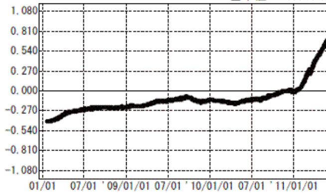
(m) (4) 硫黄島 2 (960605) → 硫黄島 1 (960604) 南北 基準値 3255.141m
