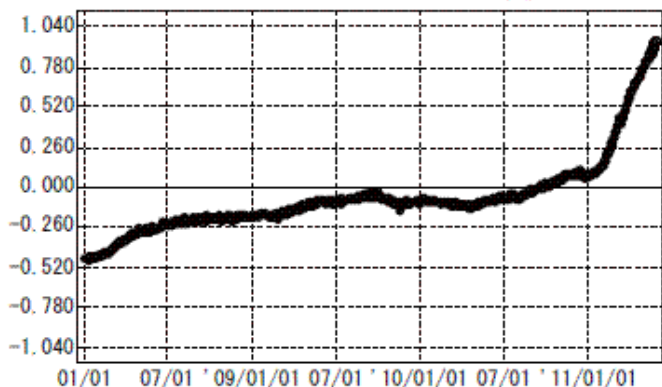
(m) (5) 硫黄島 2 (960605) → M硫黄島 (079073) 南北 基準値 3228.740m
