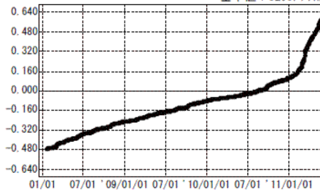
図 3※ 硫黄島 国土地理院による GPS 観測結果 1) (2008 年 1 月 1 日～2011 年 5 月 29 日)
