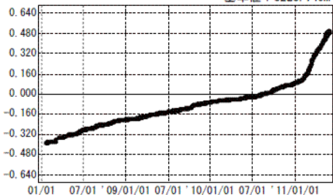
図 3※ 硫黄島 国土地理院による GPS 観測結果 1) (2008 年 1 月 1 日～2011 年 5 月 29 日)
