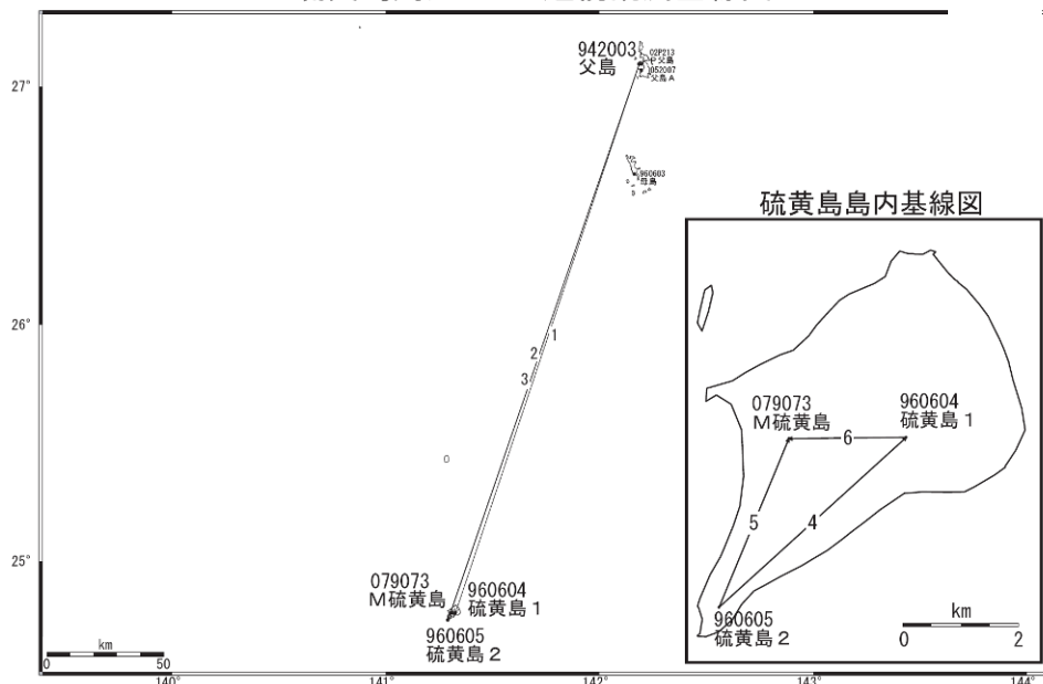
(m) (1) 父島 A (052007) → 硫黄島 1 (960604) 比高 基準値 65.815m
