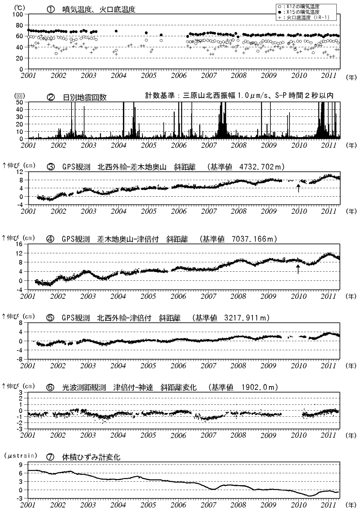
図2 伊豆大島 最近の火山活動経過図 (2001年1月～2011年4月)
