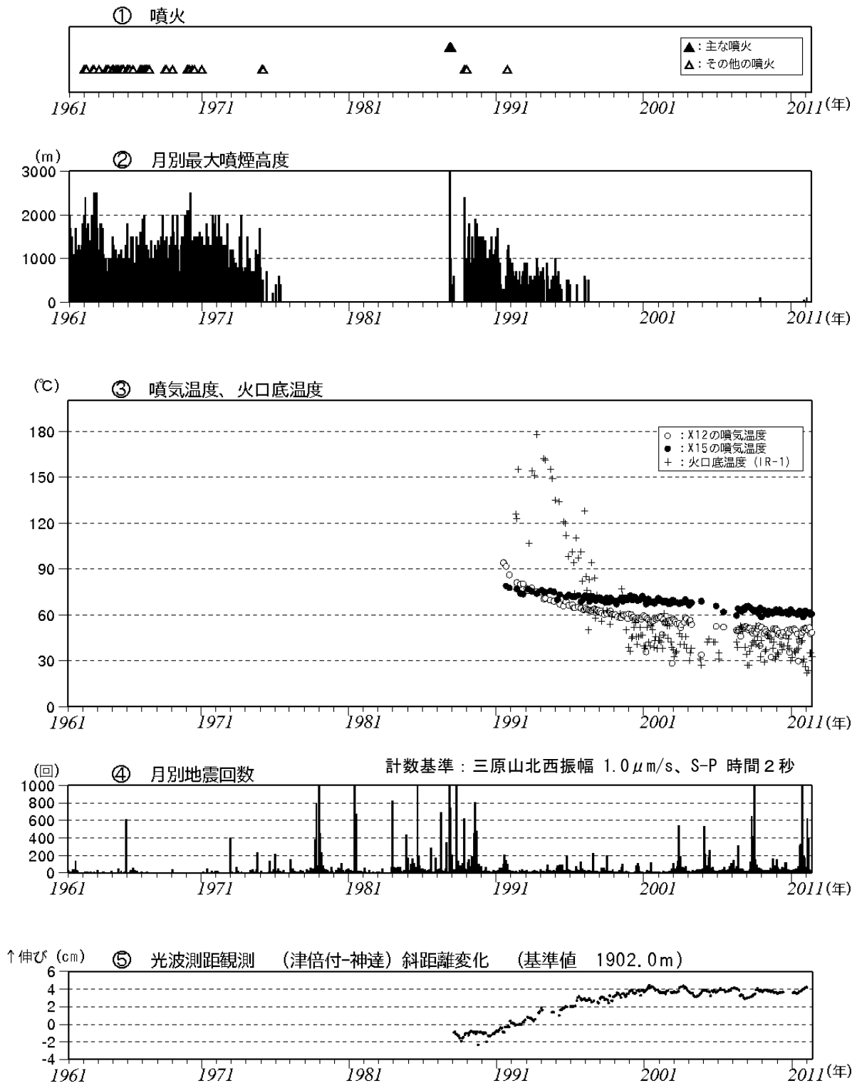
図 1 伊豆大島 長期間の火山活動経過図（1961 年 1 月～2011 年 5 月）
