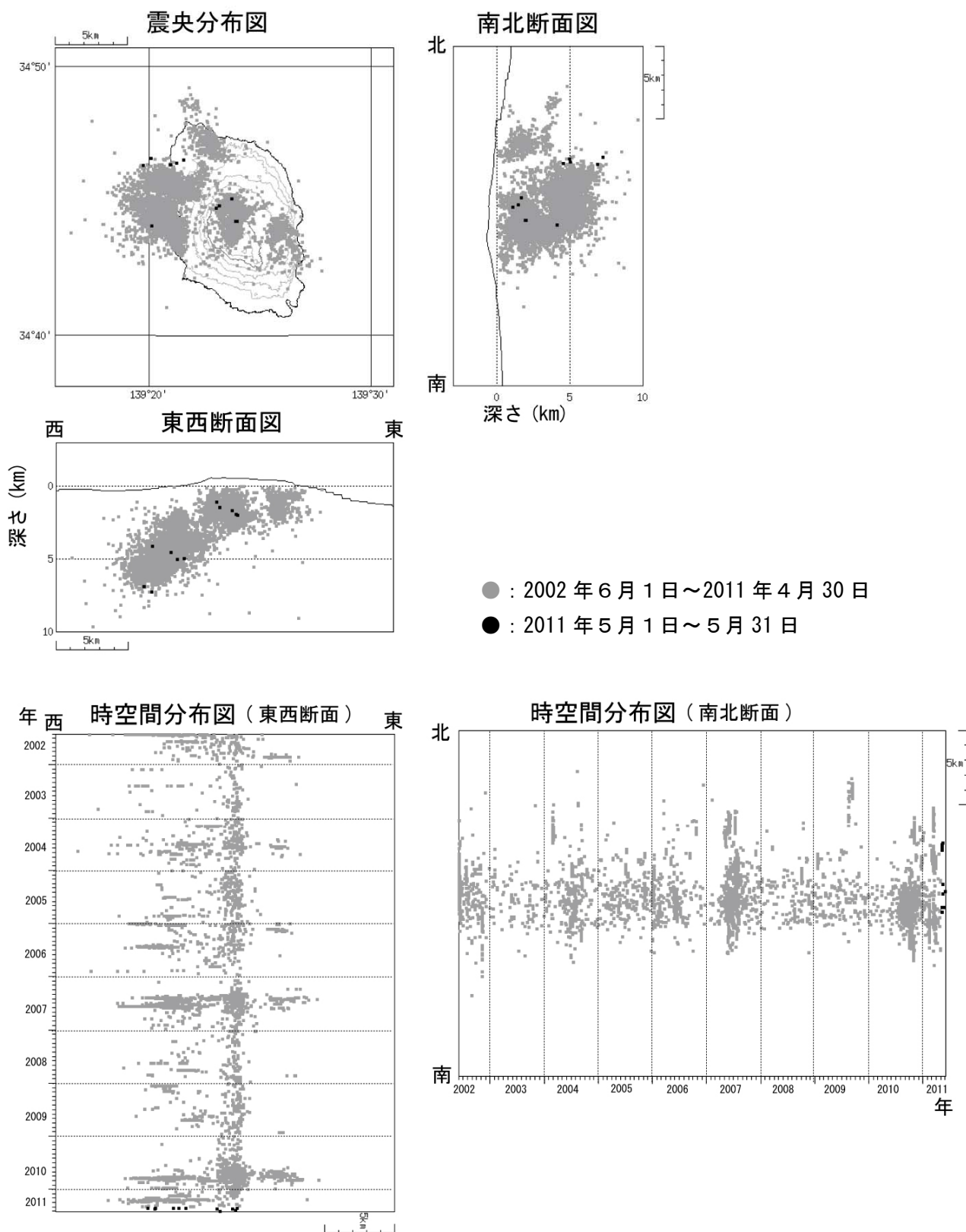
図6※ 伊豆大島 震源分布図 (2002年6月1日～2011年5月31日)
