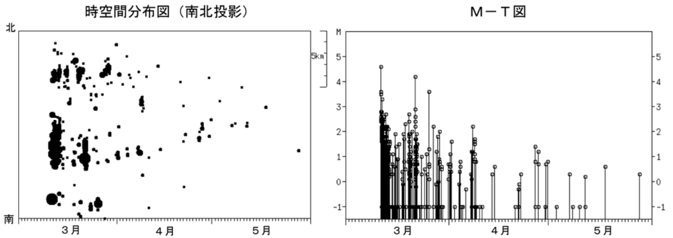
図4 箱根山 時空間分布図、M-T 図（2011 年 3 月 1 日～5 月 31 日） M（マグニチュード）は地震の規模を表します。 3～5 月分は一部未処理の期間があります。 図中の震源要素は一部暫定値が含まれており、後日変更することがあります。
