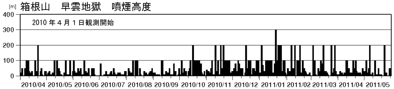
図 2 箱根山 早雲地獄の日別最大噴煙高度（2010 年 4 月 1 日～2011 年 5 月 31 日）
