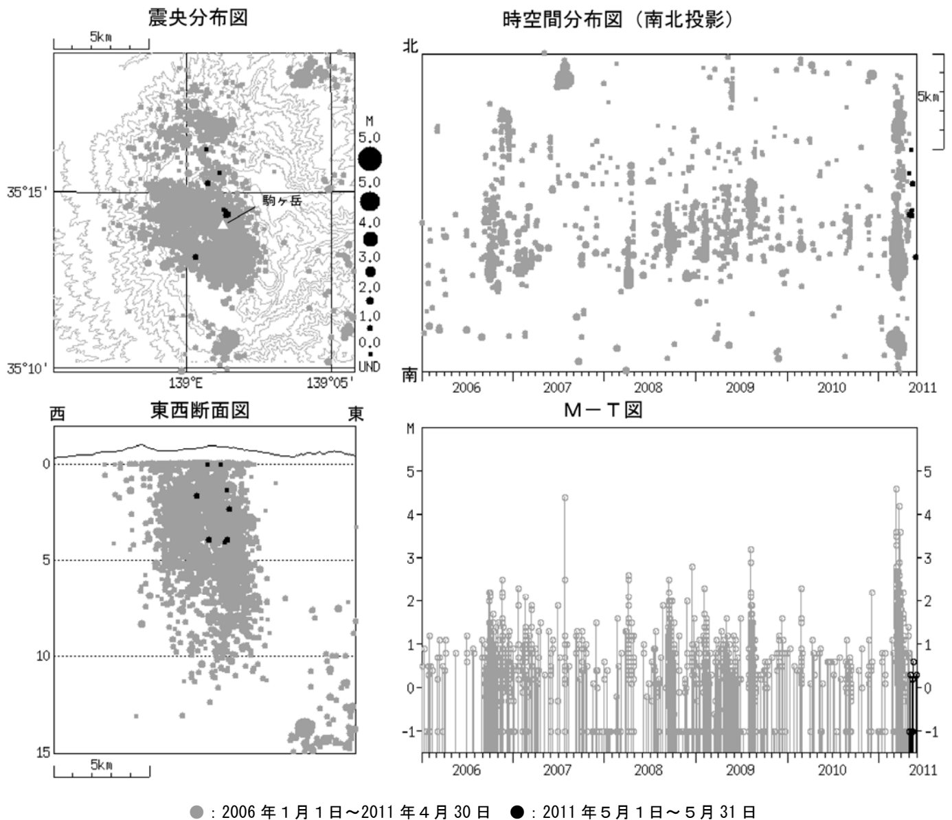
図 3 箱根山 広域ネットによる山体・周辺の震源分布図（2006 年 1 月 1 日～2011 年 5 月 31 日）
