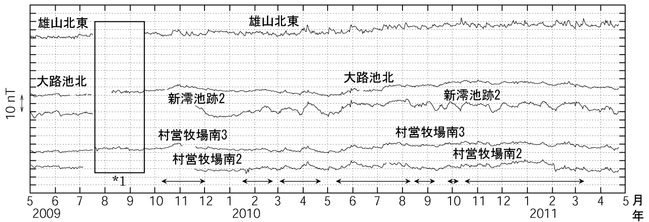
図3 三宅島 全磁力連続観測による全磁力値の変化 (2009年5月~2011年4月24日)
