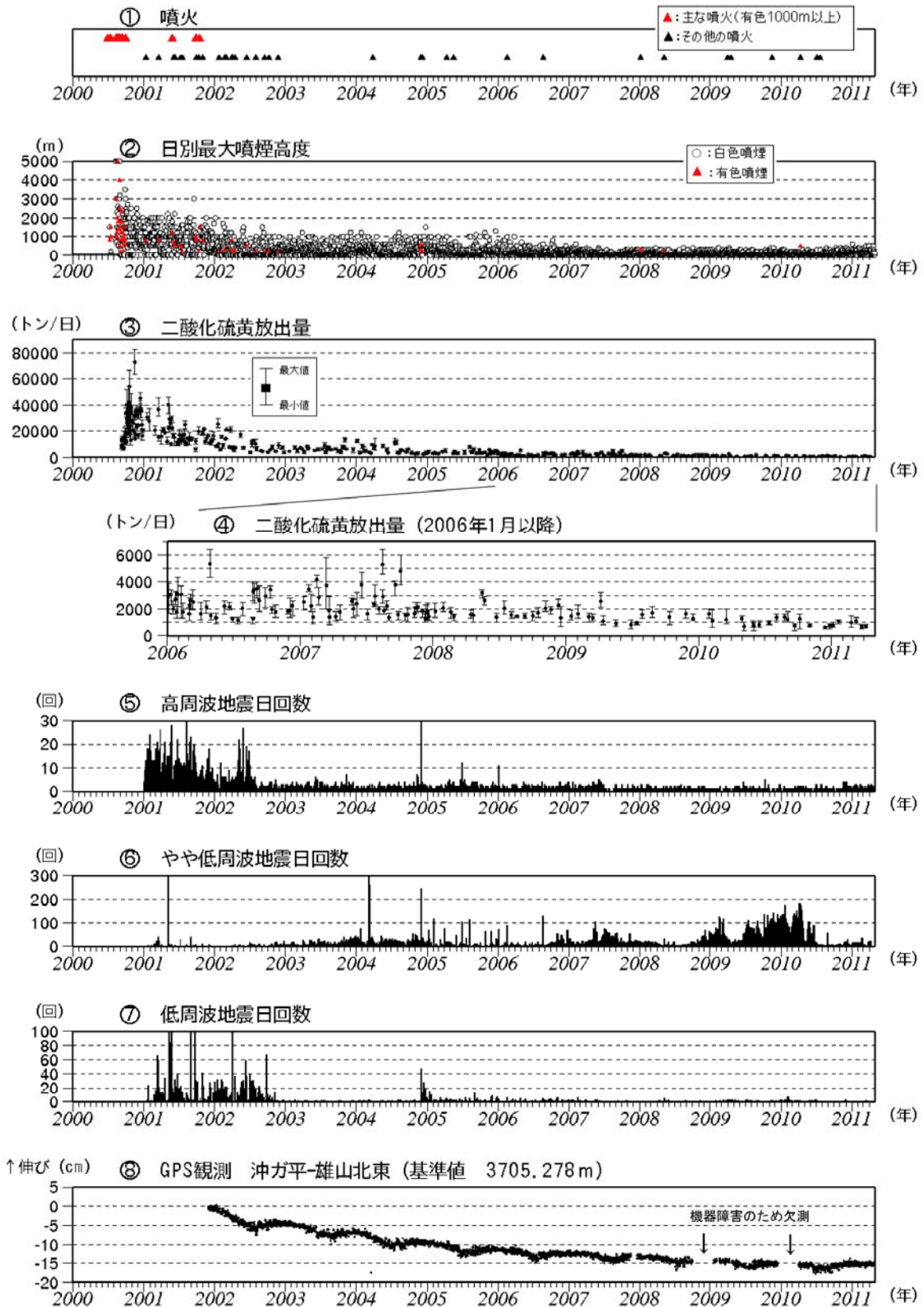
図2 三宅島 最近の火山活動の推移 (2000年1月~2011年4月)
