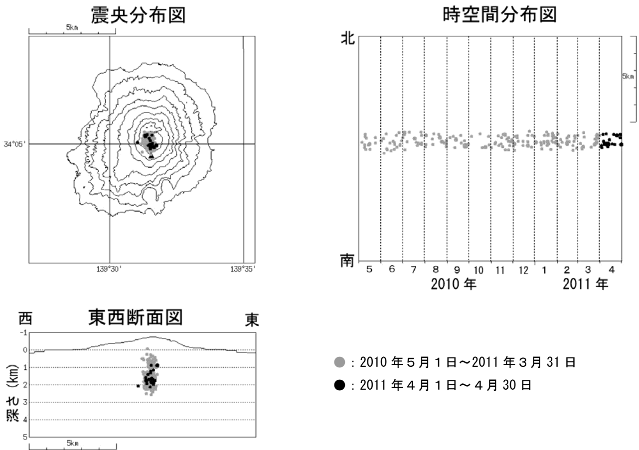
図4※ 三宅島 震源分布図 (2010年5月1日~2011年4月30日)
