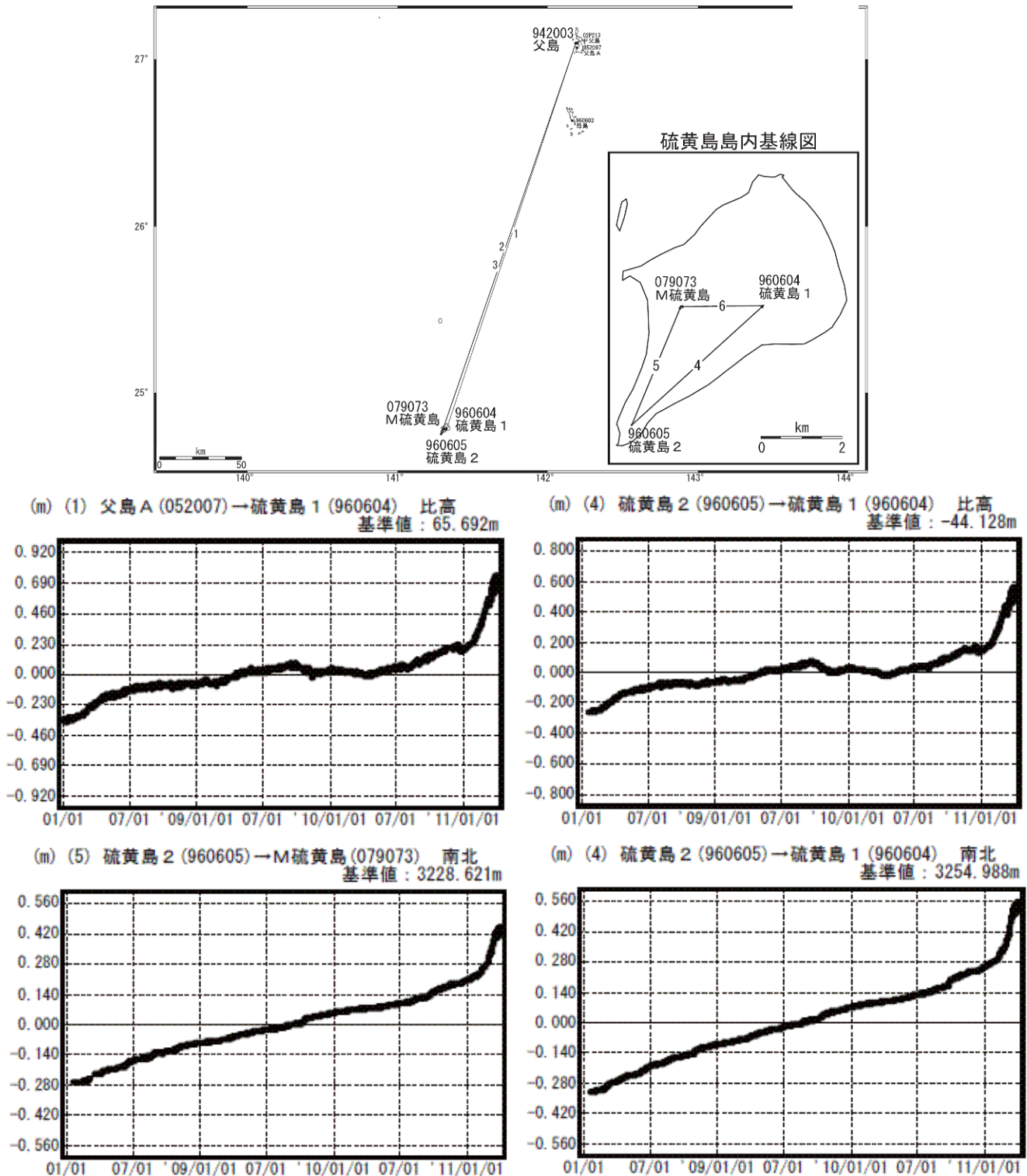
図 3※ 硫黄島 国土地理院による GPS 観測結果 1) （2008 年 1 月 1 日～2011 年 4 月 2 日）
