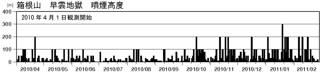
図 2 箱根山 早雲地獄の日別最大噴煙高度（2010 年 4 月 1 日～2011 年 2 月 28 日）
