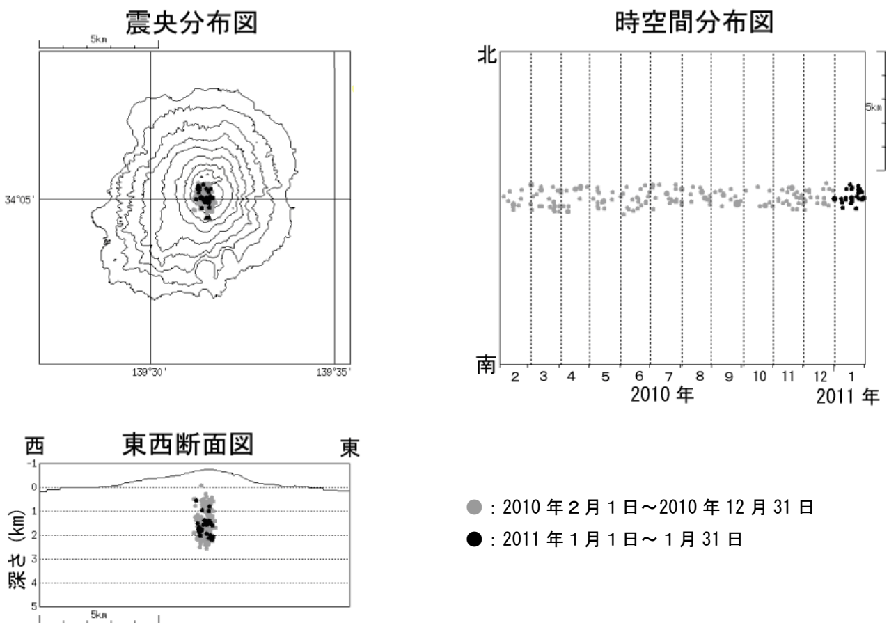
図4※ 三宅島 震源分布図 (2010年2月1日~2011年1月31日)
