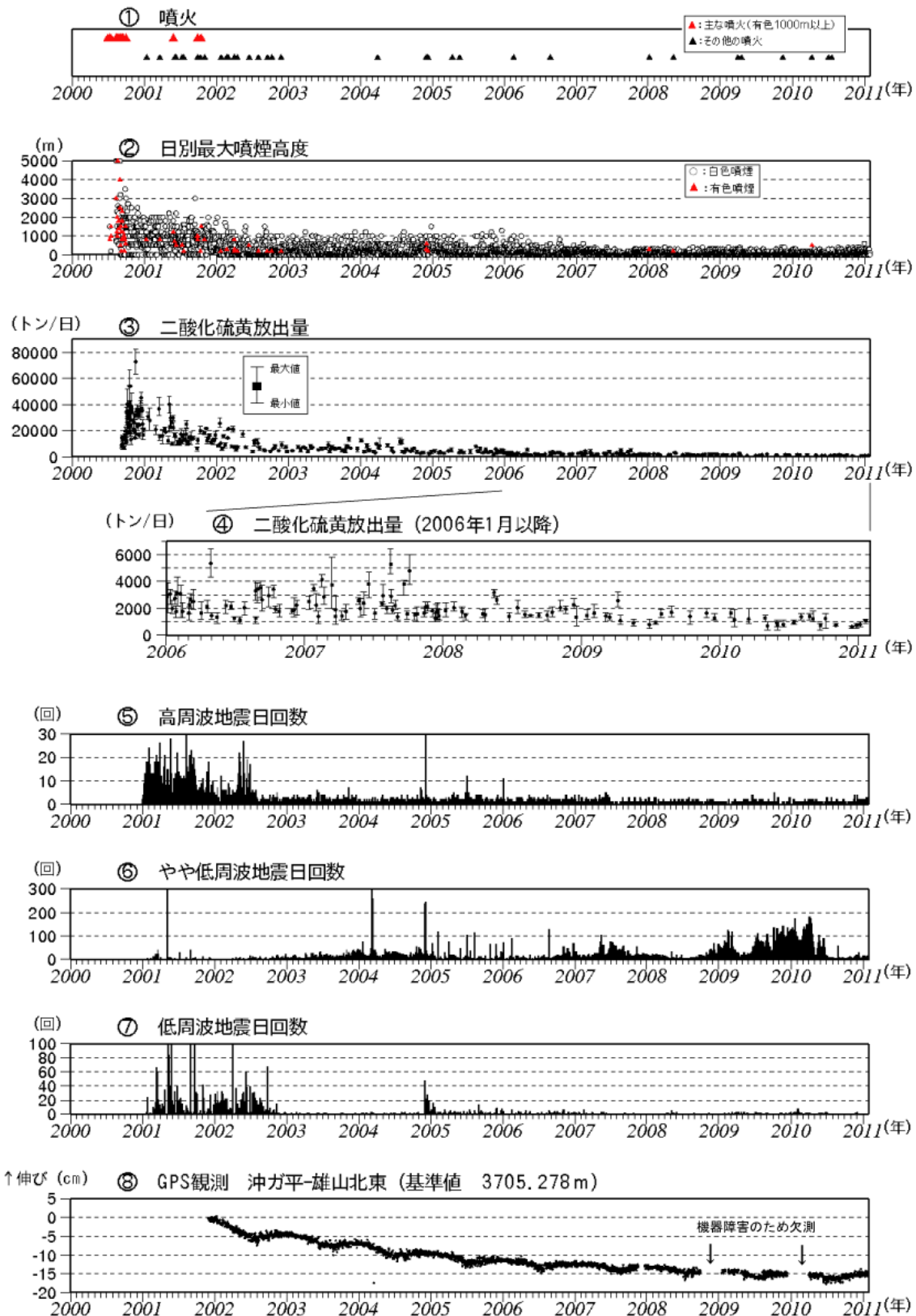
図 2 三宅島 最近の火山活動の推移（2000 年 1 月～2011 年 1 月）
