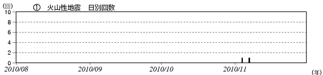
図 3 青ヶ島 火山性地震日別回数（2010 年 8 月 1 日～2010 年 11 月 30 日）
