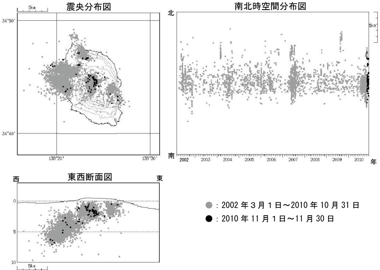
図 6※ 伊豆大島 震源分布図 (2002 年 3 月 1 日~2010 年 11 月 30 日)
