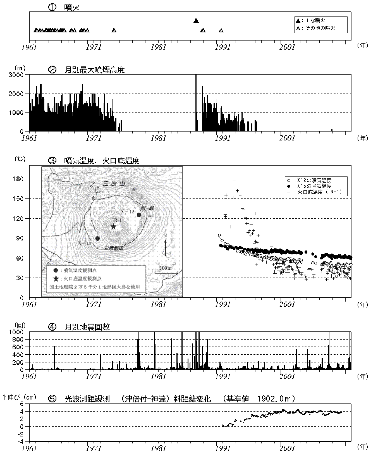
図 1 伊豆大島 長期間の火山活動経過図 (1961 年 1 月～2010 年 11 月)
