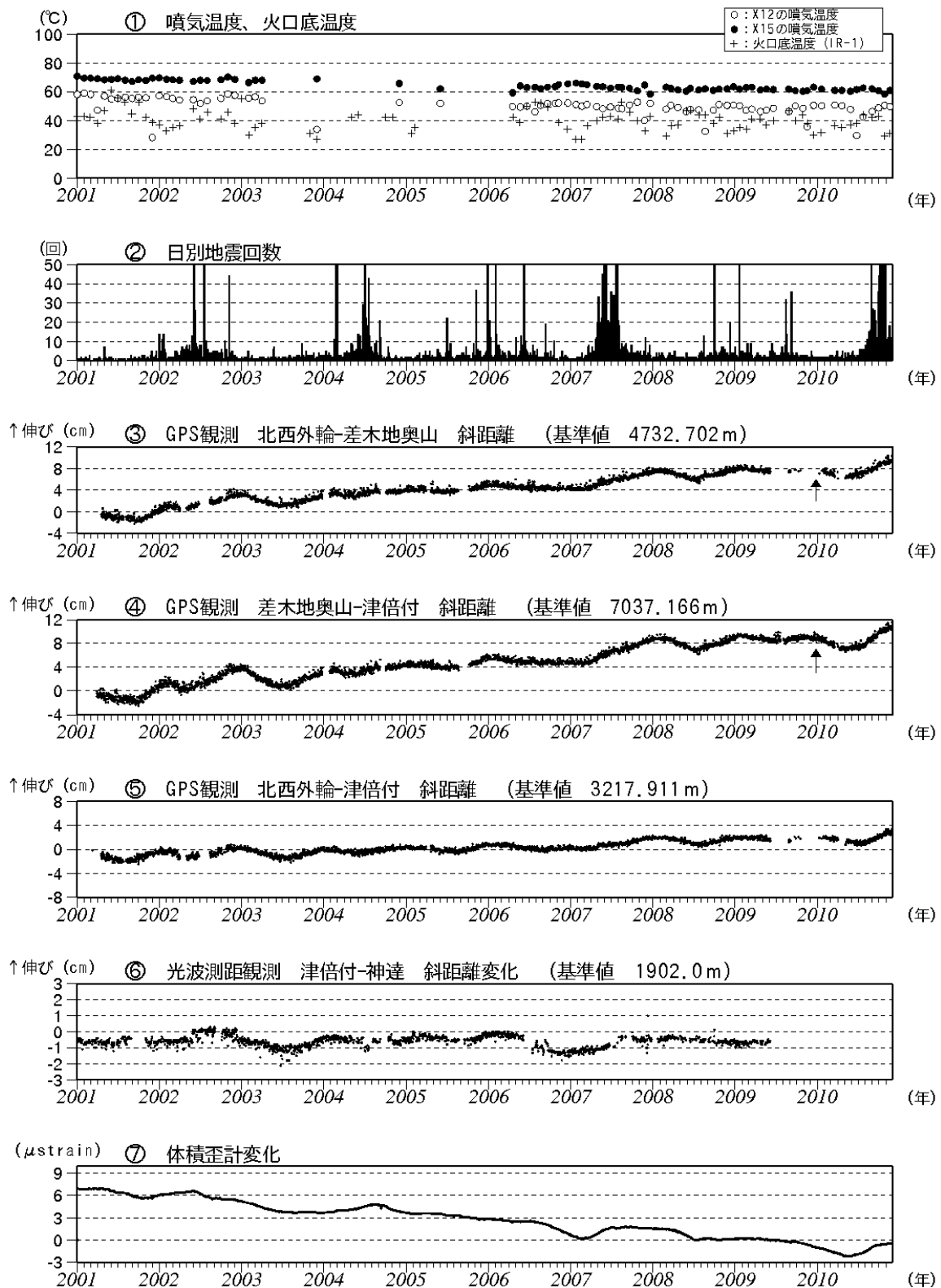
図2 伊豆大島 最近の火山活動経過図 (2001年1月～2010年11月)
