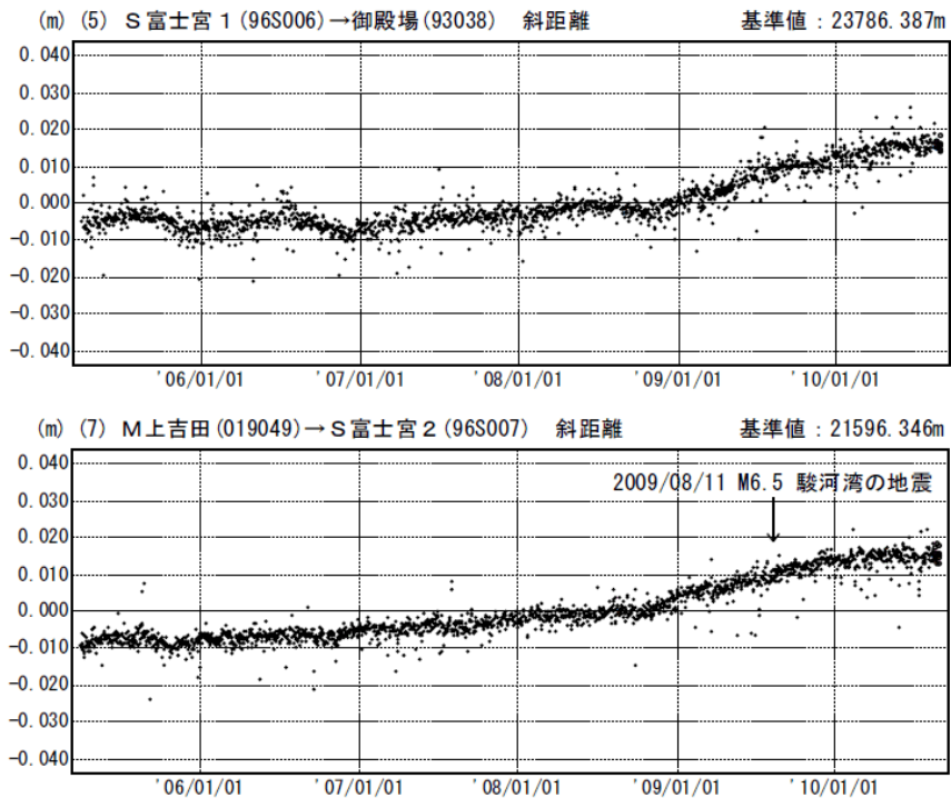
図 3※ 富士山 国土地理院による GPS 観測結果 1) （2005 年 4 月 1 日～2010 年 8 月 29 日）
