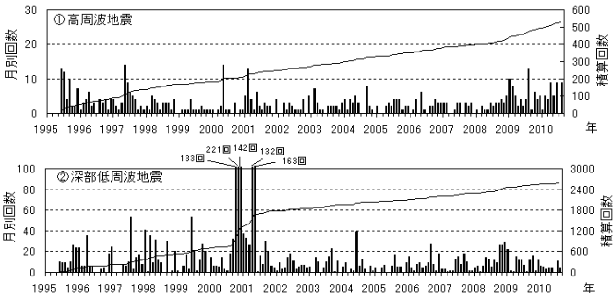
図 1※ 富士山 月別地震回数(1995 年 6 月～2010 年 8 月)
