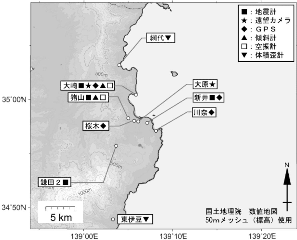
図 5 伊豆東部火山群 新しい観測点名称を使用した観測点配置図 （小さな白丸は気象庁の観測点位置を示しています） 運用開始前の観測点も含まれます。
