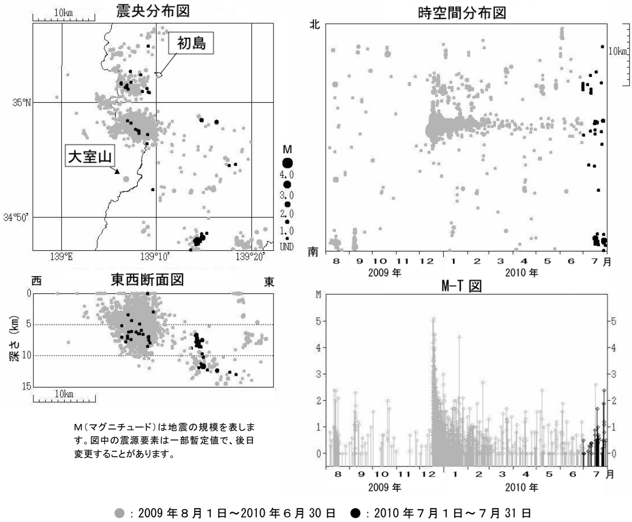
図 2 ※ 伊豆東部火山群 震源分布図 (2009 年 8 月 1 日 ~ 2010 年 7 月 31 日)
