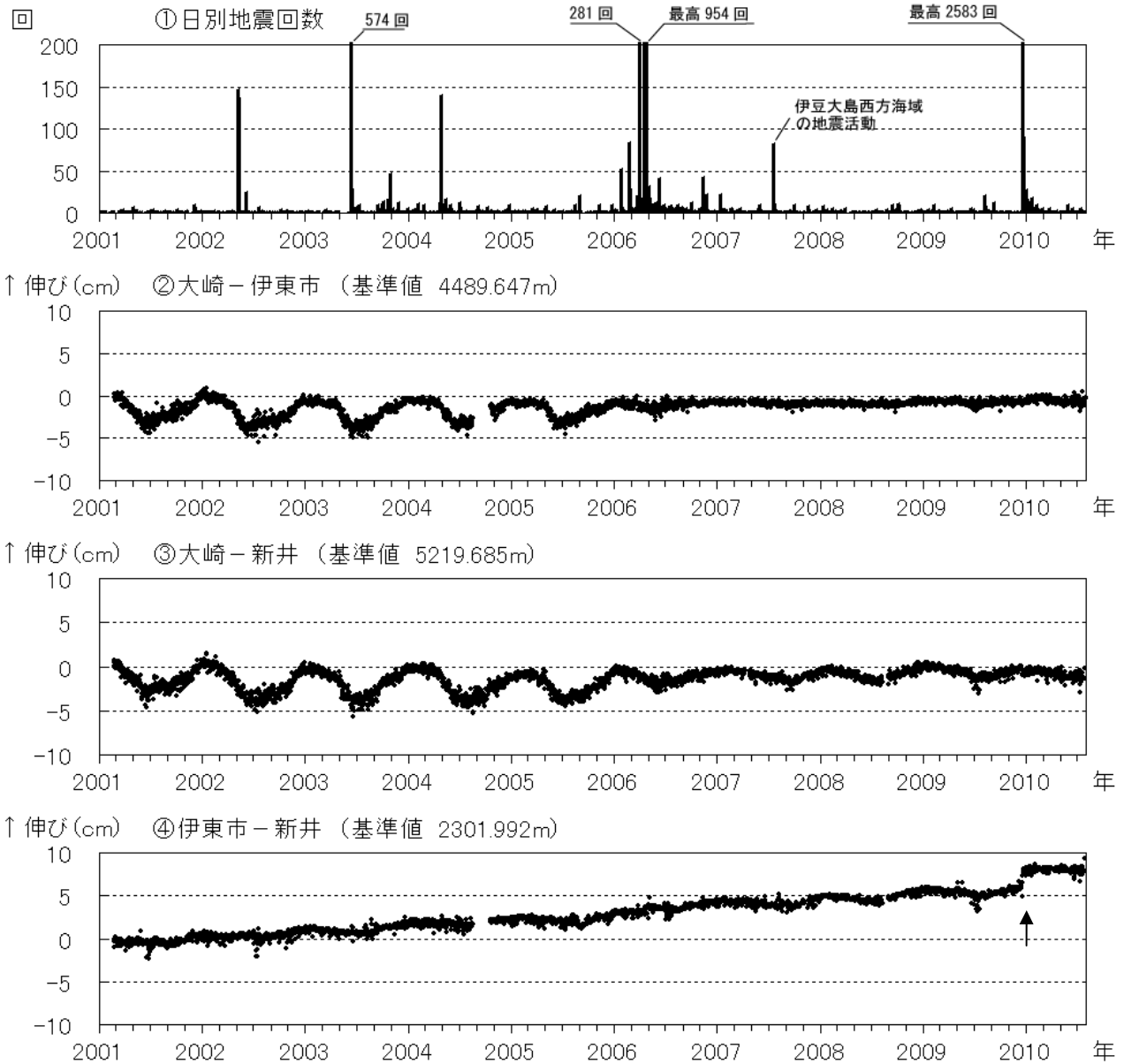
図 3 伊豆東部火山群 最近の火山活動の推移（2001 年 1 月～2010 年 7 月）
