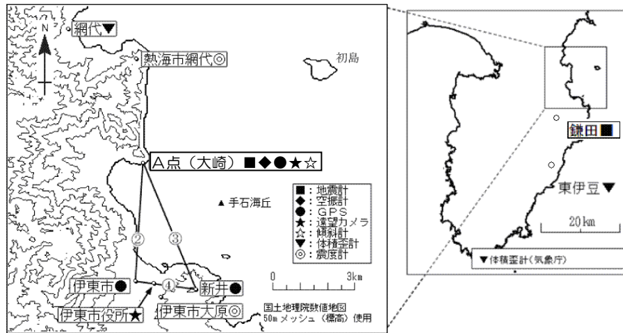
図4 伊豆東部火山群 気象庁の観測点配置図（小さな白丸は観測点位置を示しています） GPS基線②～④は図3の②～④に対応しています。
