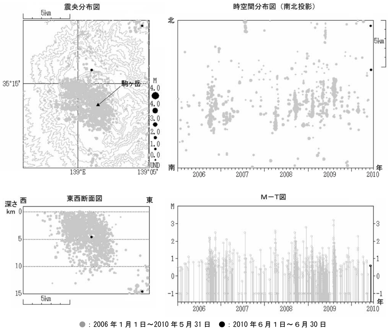
図 5※ 箱根山 震源分布図（2006 年 1 月 1 日～2010 年 6 月 30 日） M（マグニチュード）は地震の規模を表します。 図中の震源要素は一部暫定値が含まれており、後日変更することがあります。
