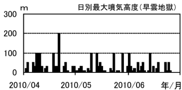
図 4 早雲地獄の日別最大噴気高度
