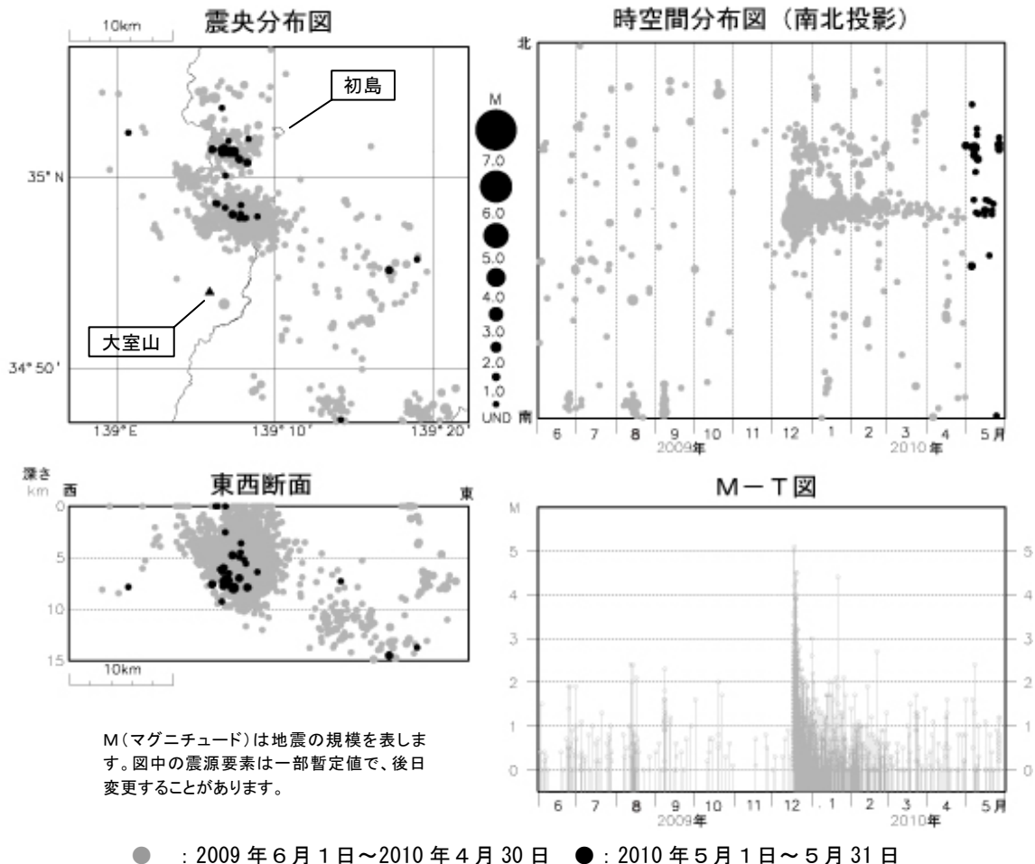
図 1※ 伊豆東部火山群 震源分布図（2009 年 6 月 1 日～2010 年 5 月 31 日）
