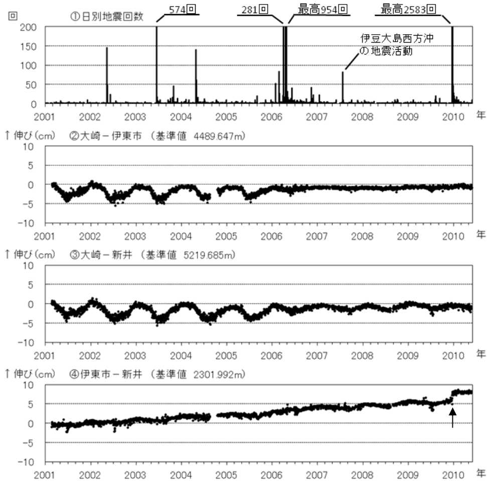
図 2 伊豆東部火山群 最近の火山活動の推移 (2001 年 1 月～2010 年 5 月)
