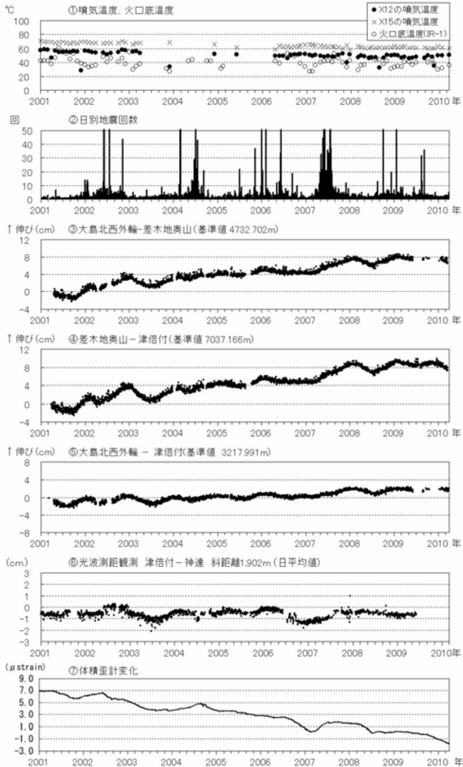
図5 伊豆大島 最近の火山活動経過図(2001年1月~2010年3月)
