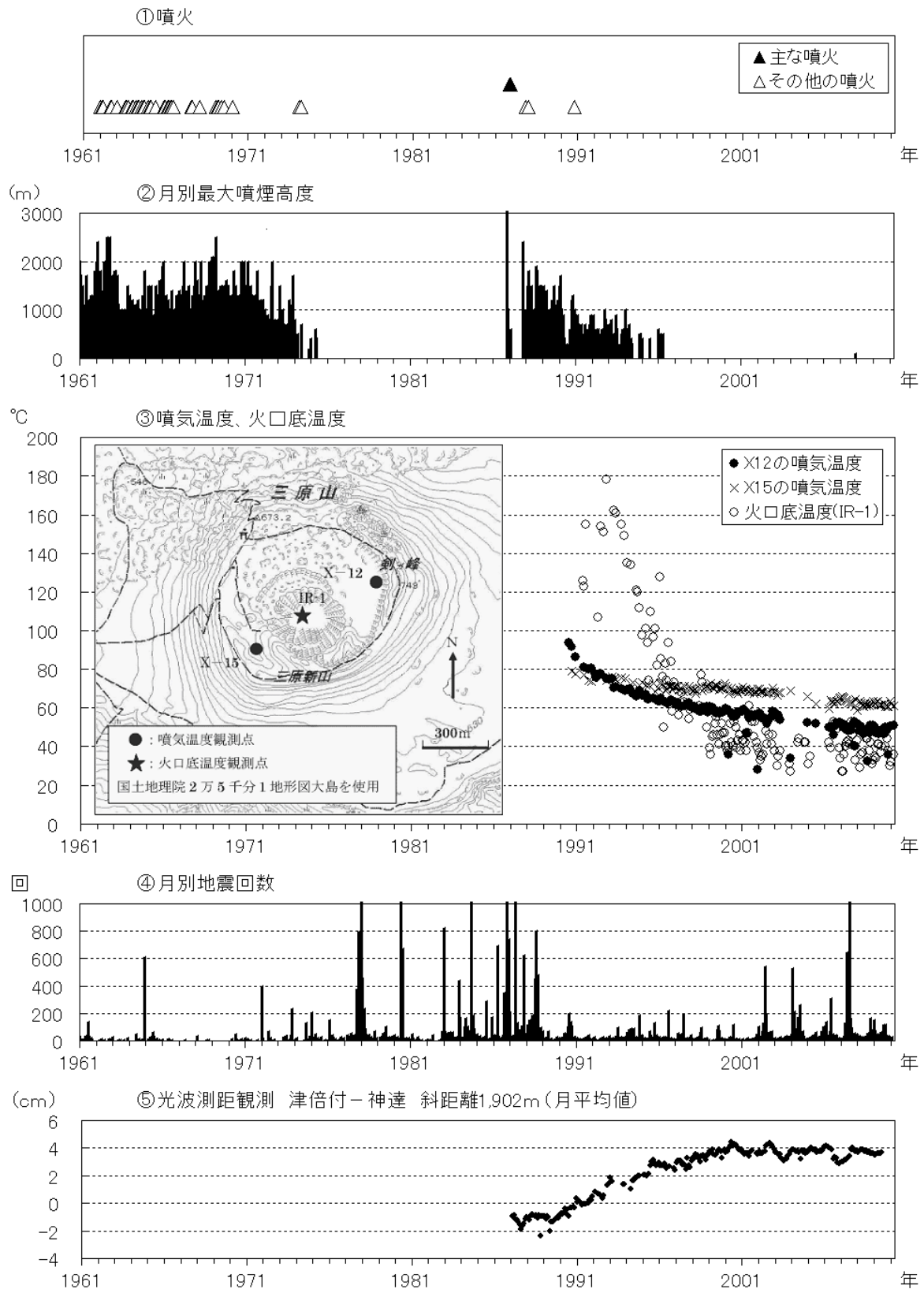
図4 伊豆大島 長期間の火山活動経過図（1961年1月～2010年3月）
