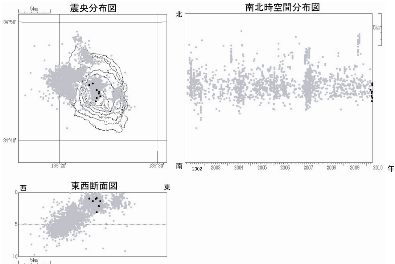
図 6 伊豆大島 震源分布図（2002 年 3 月 1 日 ~ 2010 年 3 月 31 日）
