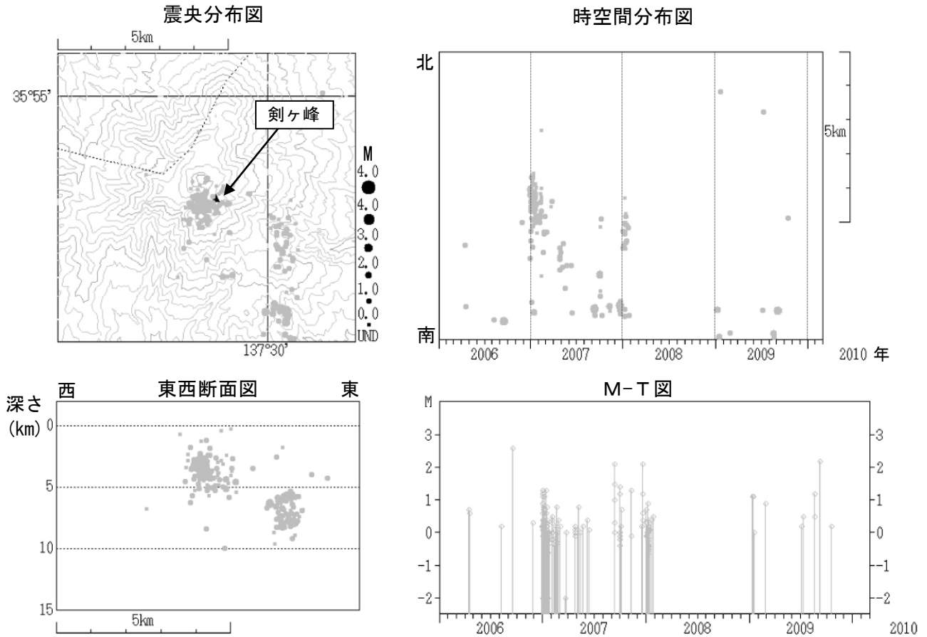
図 3※ 御嶽山 震源分布図（2006 年 1 月 1 日～2010 年 2 月 28 日）
