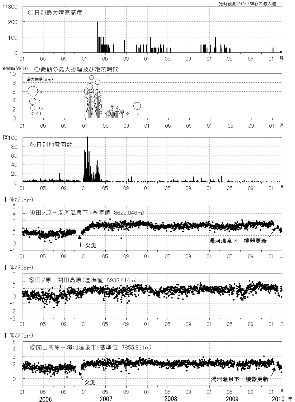
図 2 御嶽山 最近の火山活動の推移（2006 年 1 月 1 日～2010 年 2 月 28 日）
