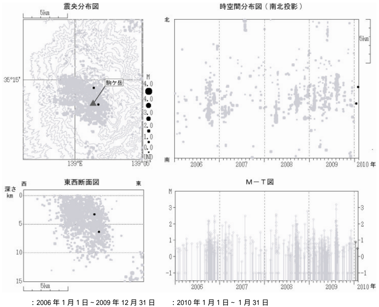
図 3 箱根山 震源分布図（2006年1月1日～2010年1月31日） M（マグニチュード）は地震の規模を表します。 図中の震源要素は一部暫定値が含まれており、後日変更することがあります。
