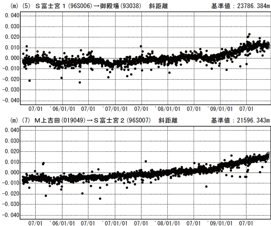
図3 富士山 国土地理院によるGPS観測結果 1) (2005年4月1日~2009年11月30日)
