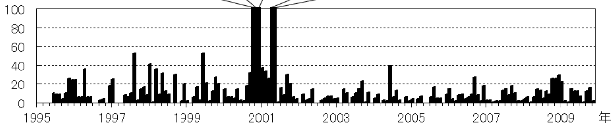
図 2 富士山 月別地震回数(1995 年 6 月 ~ 2009 年 11 月)
