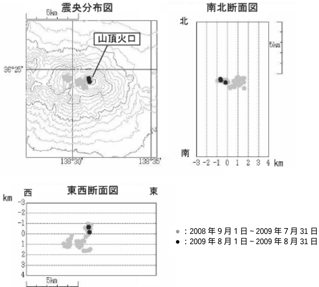
図 4 浅間山 震源分布図（2008 年 9 月 1 日～2009 年 8 月 31 日）
