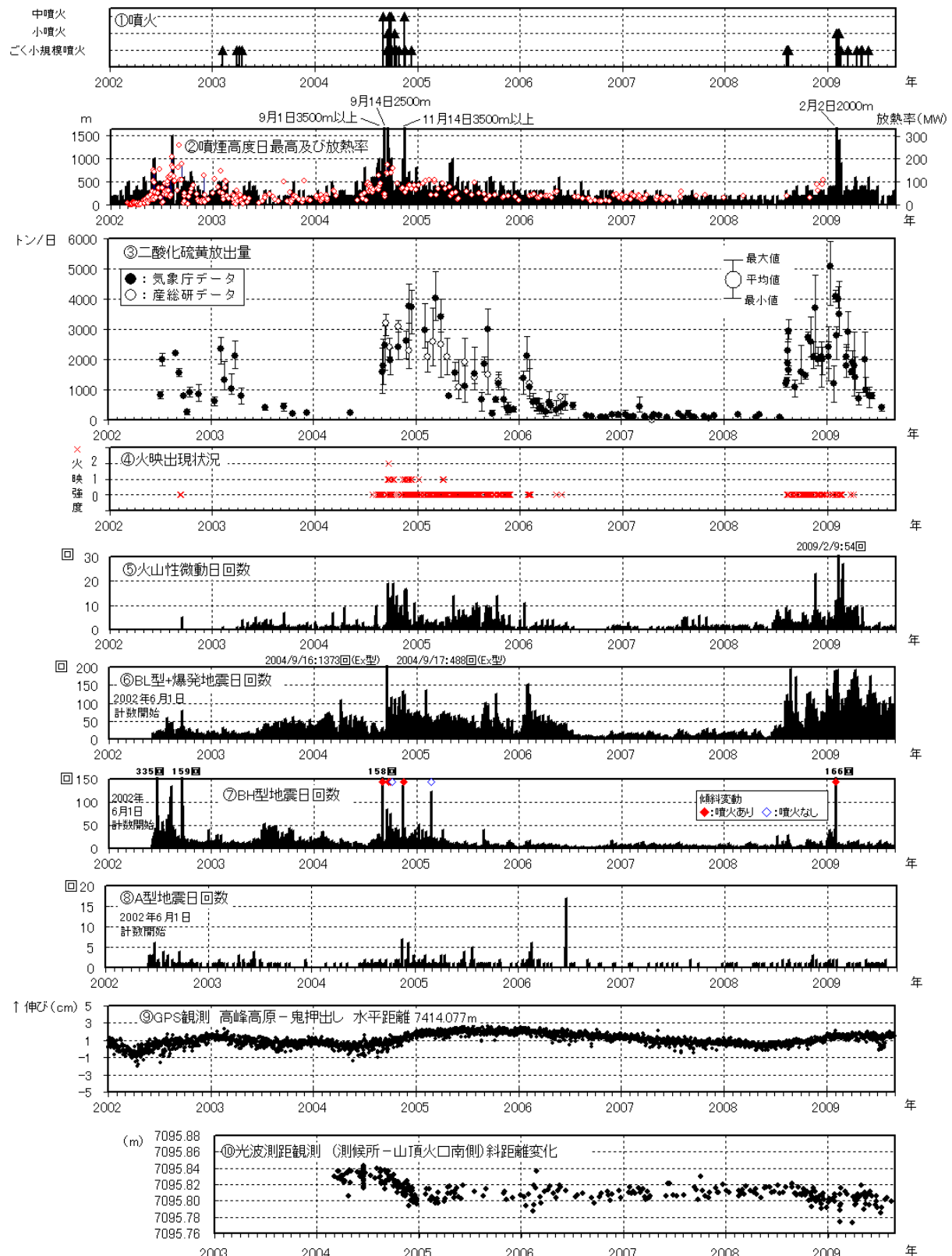
図3 浅間山 最近の火山活動の推移（2002年1月1日～2009年8月31日）
