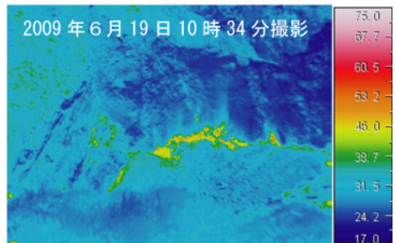
図2 伊豆大島 中央火口内の状況（左）と地表面温度分布 1) （右） （左の写真の白枠部分が右の赤外熱映像撮影部分）
