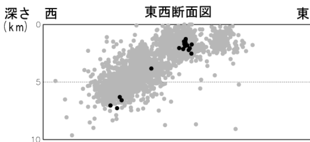
図6 伊豆大島 震源分布図(2002年3月1日~2009年6月30日)
