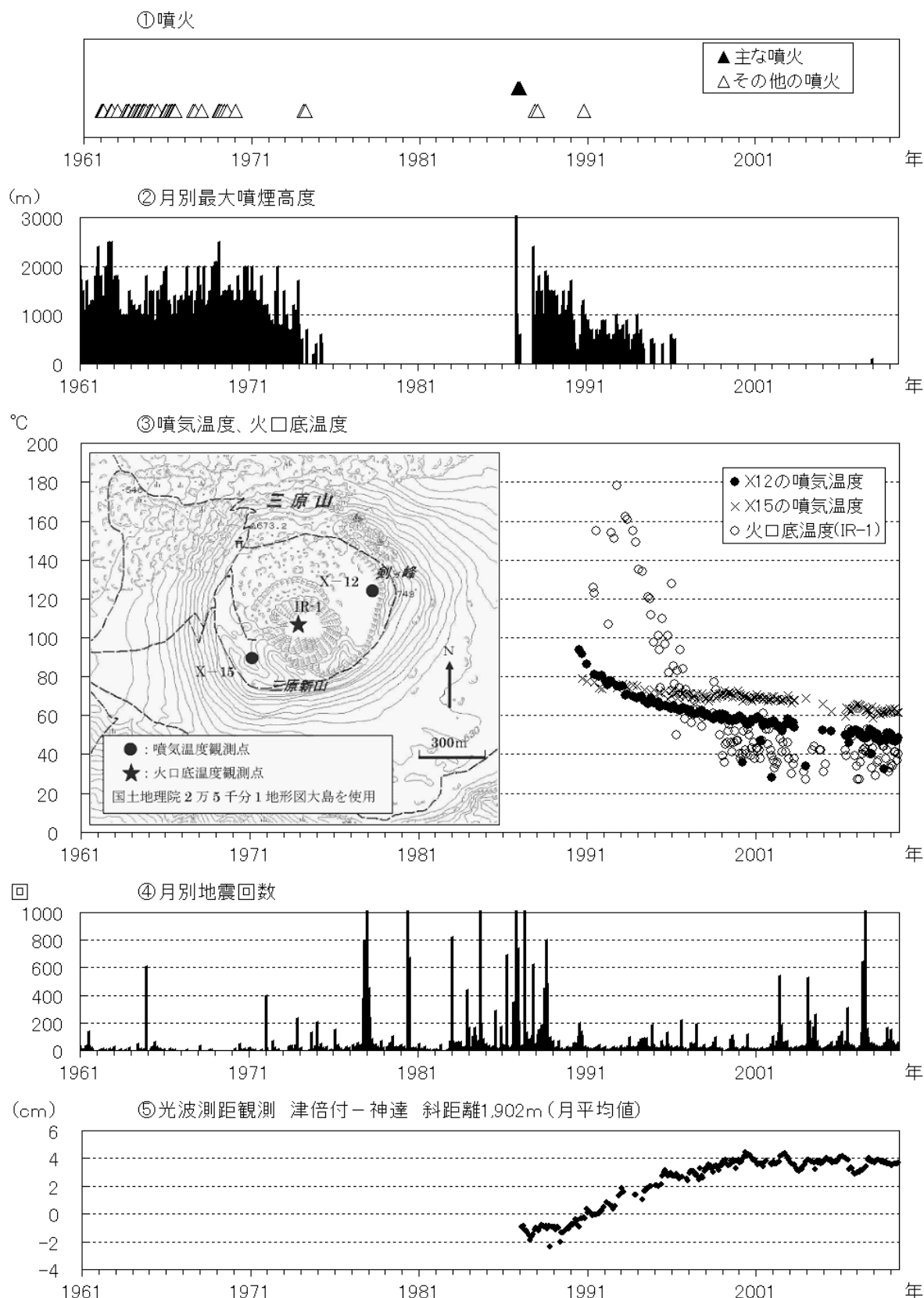
図4 伊豆大島 長期間の火山活動経過図（1961年1月～2009年6月） 1991年12月18日までは火口縁上130m以上、2002年2月28日までは火口縁上300m以上の噴煙高度を観測していました。 火口底温度（IR-1）は赤外放射温度計 1) を用いて離れた場所（図3赤外熱映像観測点と同じ）から測定した値。噴気温度（X-12、X-15）はサーミスタ温度計を用いて直接測定した値。 地震回数には伊豆大島周辺海域で発生した地震も一部含まれています。 光波距離計 2) による月平均値（観測開始は1987年1月）。
