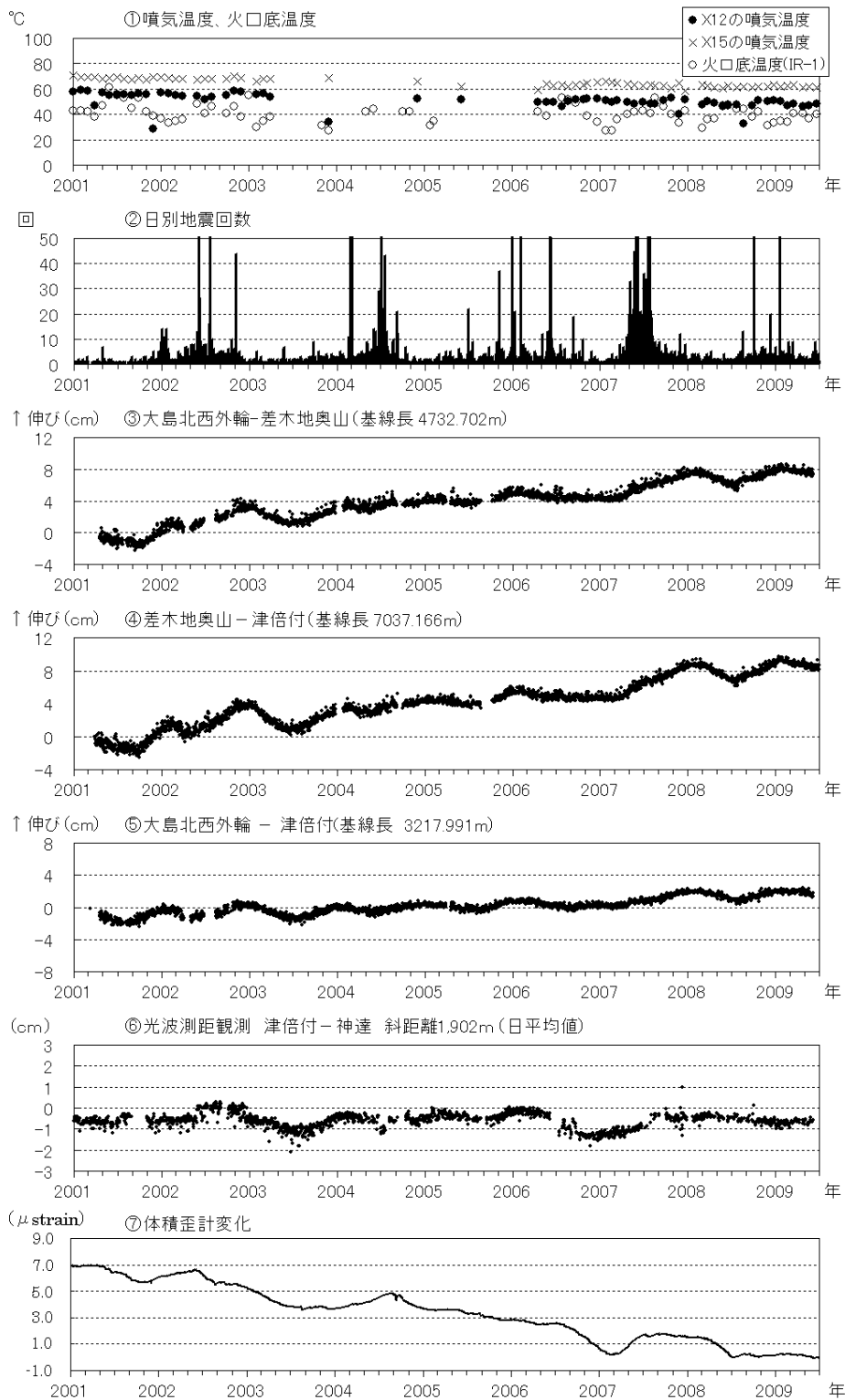
図5 伊豆大島 最近の火山活動経過図(2001年1月~2009年6月)
