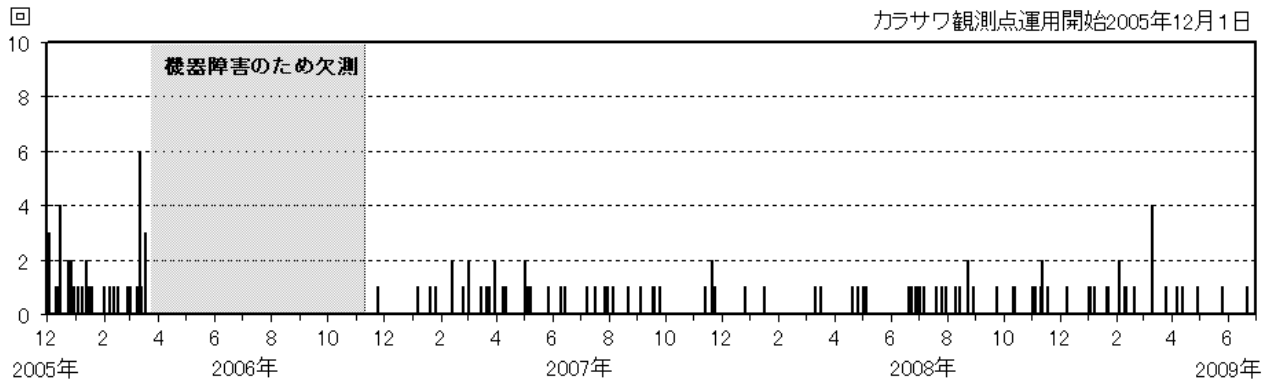
図2 新潟焼山 日別地震回数（2005年12月1日～2009年6月30日）
