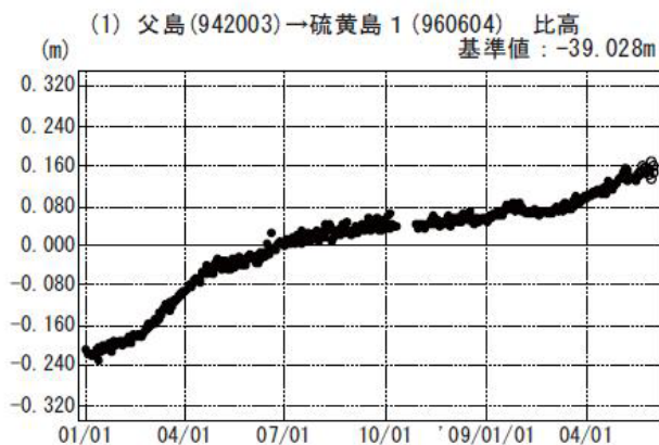
図 1 硫黄島 国土地理院による GPS 観測結果 1) (2008 年 1 月 1 日 ~ 2009 年 5 月 31 日)
