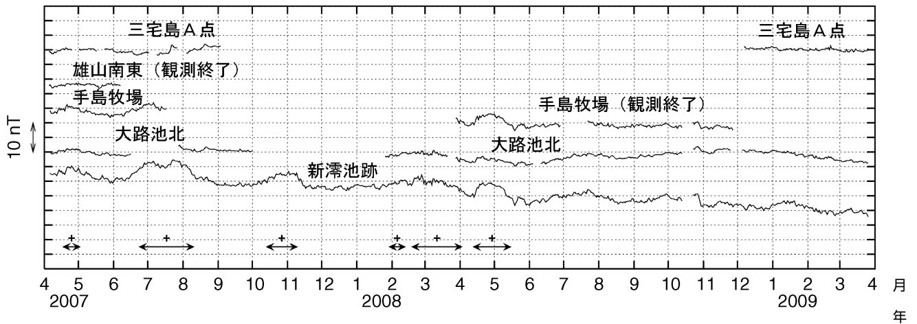
図5 三宅島 全磁力連続観測による全磁力値の変化(2007年4月~2009年3月29日) ←→ で示した期間の全磁力値は三宅島周辺の海流の影響を受けていると推測されます。 nT(ナノテスラ)は磁場の強さを表す単位です。 2008年10月下旬の全磁力減少の原因は不明ですが、黒潮の流軸が離れていく場合に同様の傾向がみられます。
