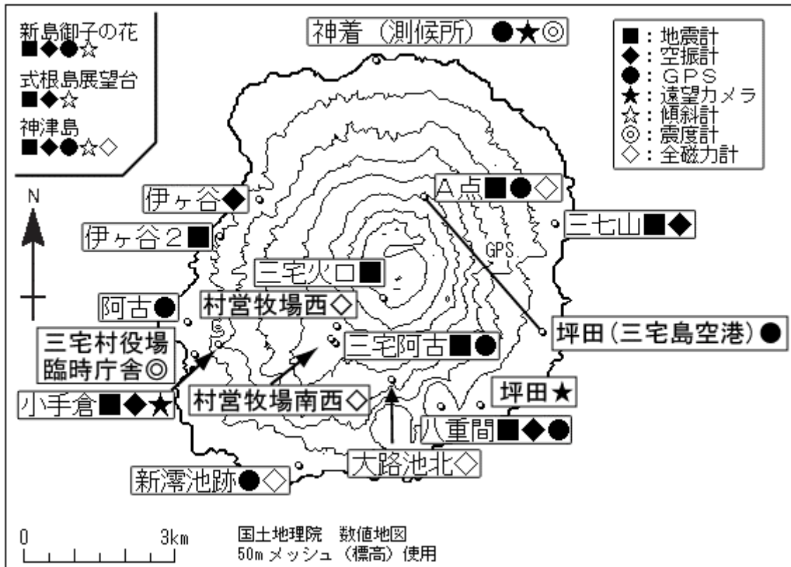
図 8 三宅島 気象庁の観測点配置図（小さな白丸は観測点位置を示しています） GPS 基線（A点 - 坪田）は図 2 の に対応しています。
