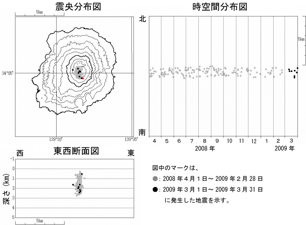
図6 三宅島 震源分布図(2008年4月1日~2009年3月31日)
