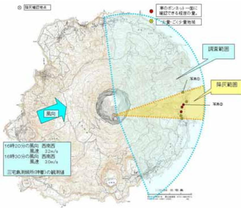
図2 降灰調査結果
