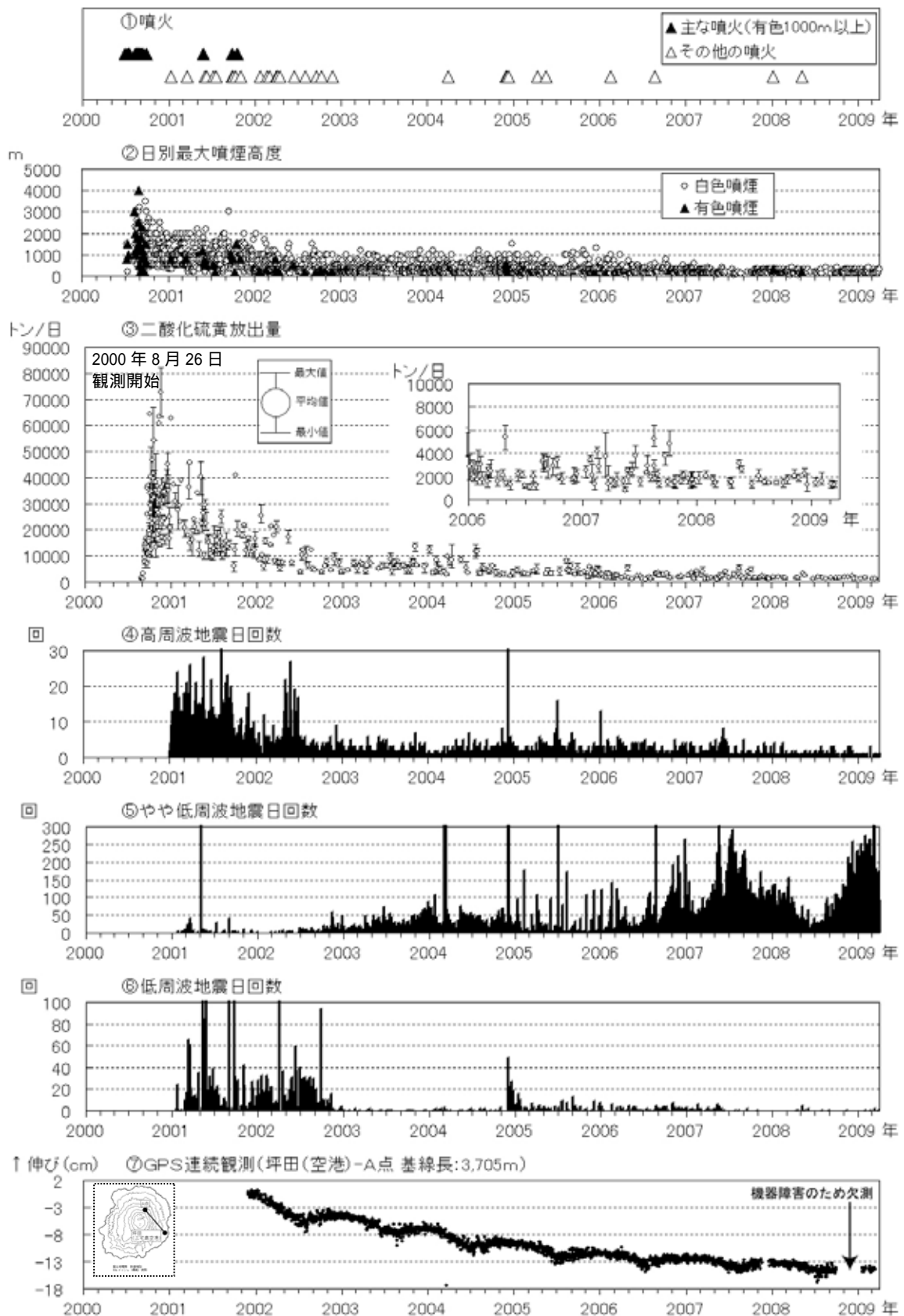
図4 三宅島 最近の火山活動の推移（2000年1月～2009年3月）
